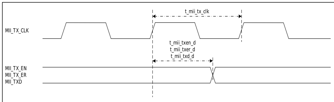
图 3-20 ETHMAC-MII 接口输出信号时序图
