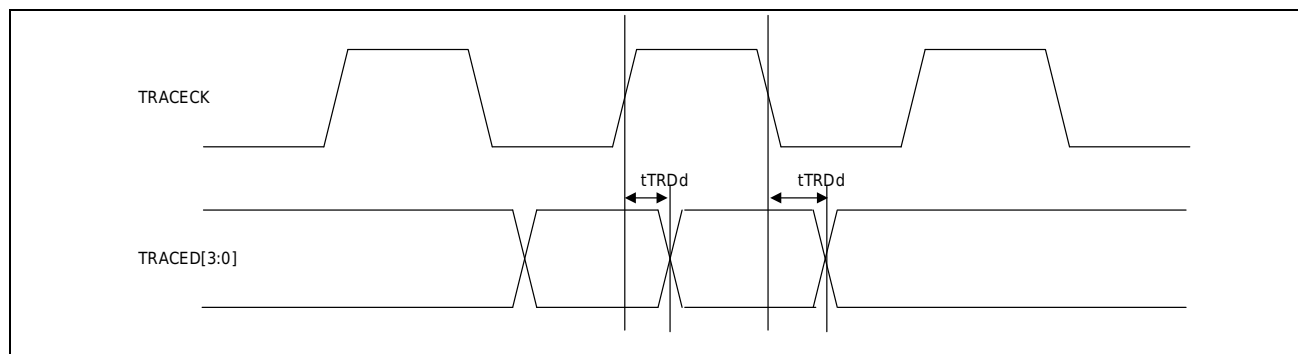
图 3-30 TRACE DATA 输出
