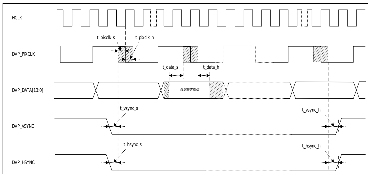
图 3-36 DVP 输入信号时序图
