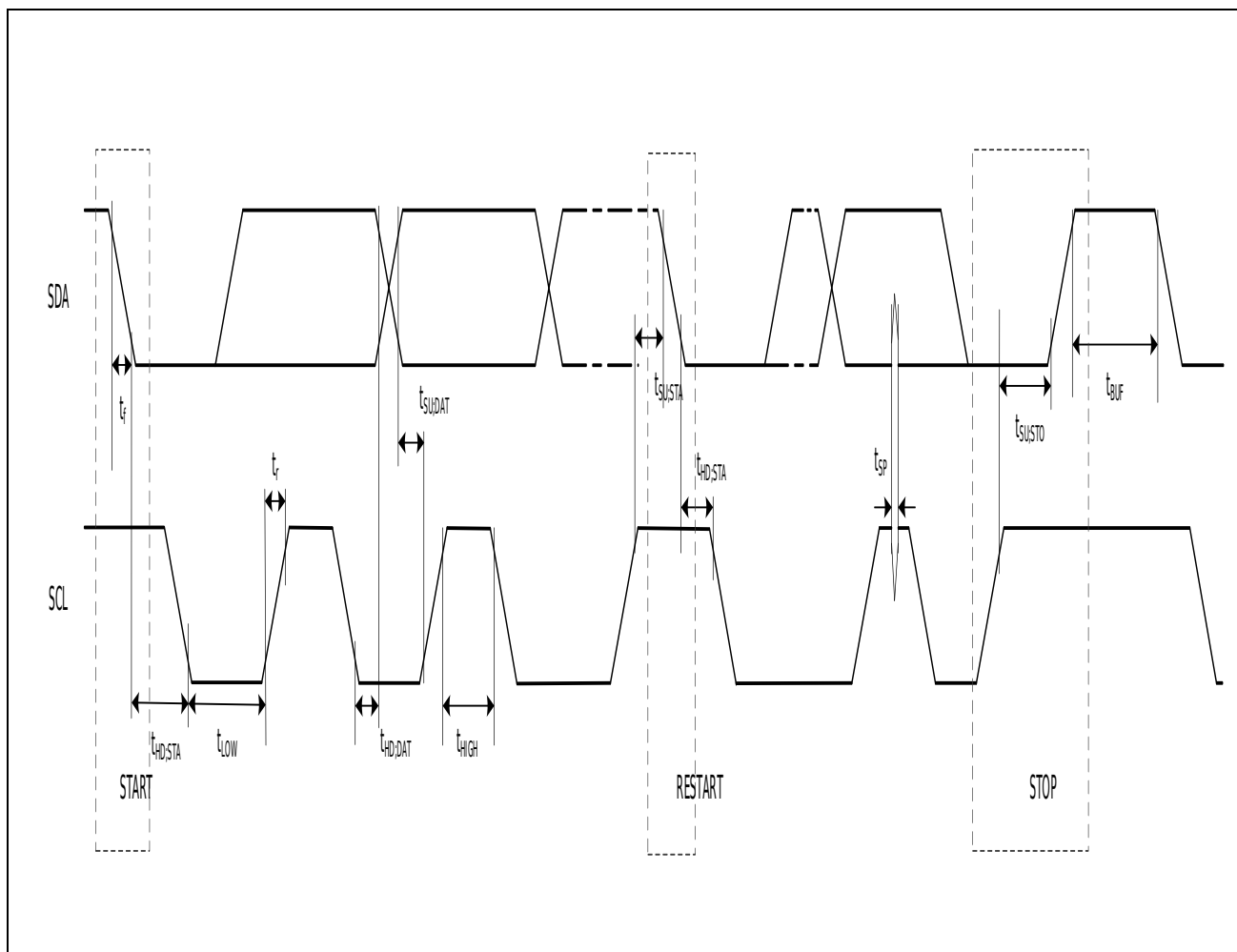
图 3-9 I2C 总线时序定义
