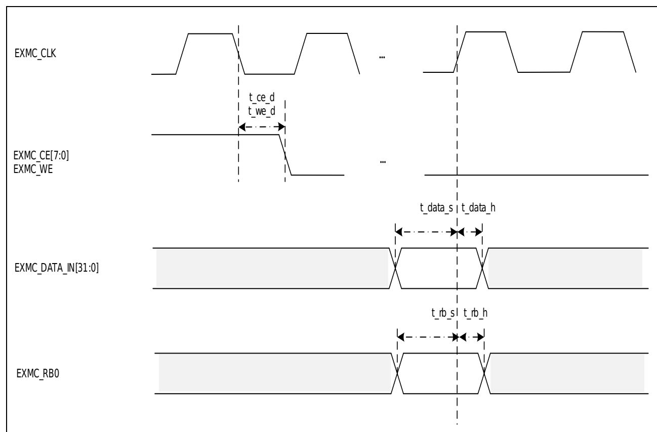
图 3-35 EXMC 输入信号时序图
