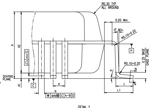
DETAIL Y
