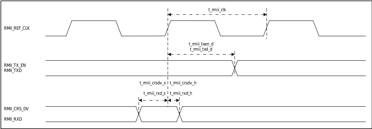
图 3-22 ETHMAC-RMII 接口时序图
