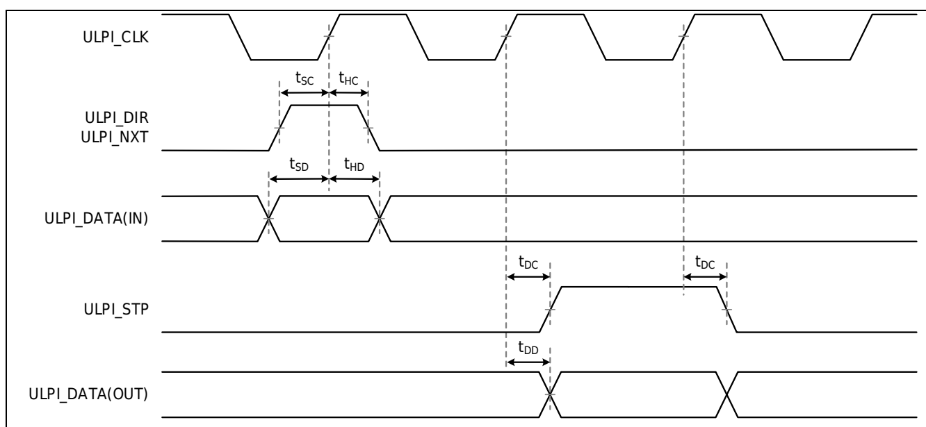
图 3-18 ULPI 时序图
