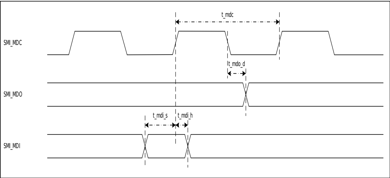
图 3-19 ETHMAC-SMI 接口时序图
