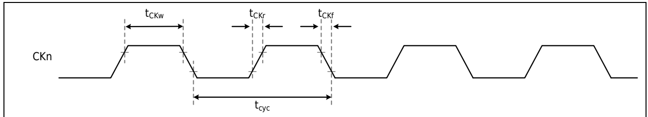
图 3-23 USART 时钟时序
