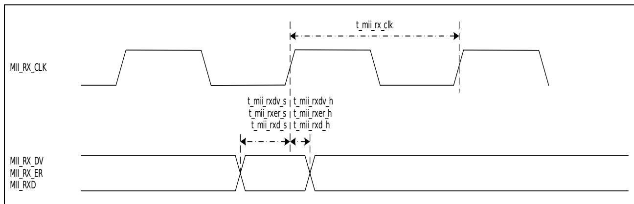
图 3-21 ETHMAC-MII 接口输入信号时序图
