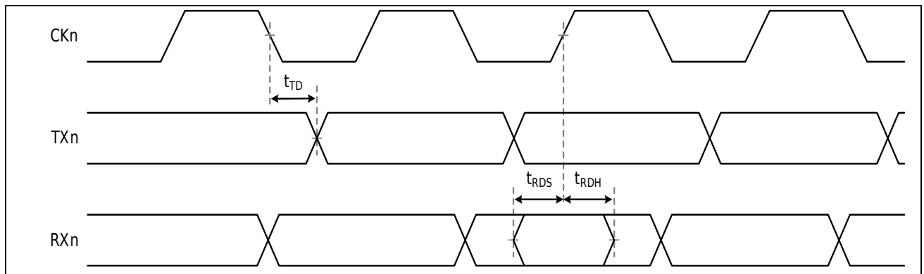
图 3-24 USART (CSI) 输入输出时序
