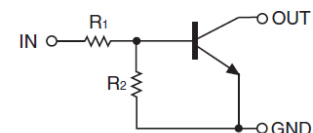
SOT-323 (USM(SC-70-3))
