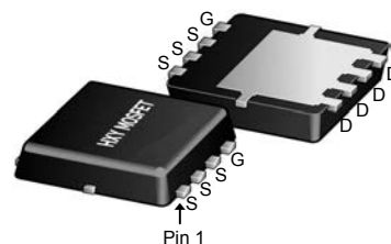
DFN5X6-8L (PowerDI5060-8)
