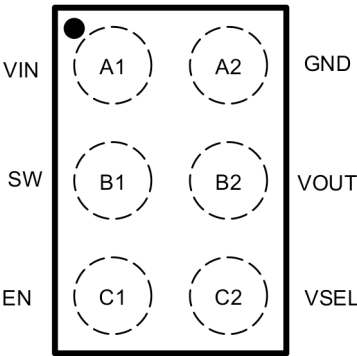
图 5-1. YBH 封装顶视图
