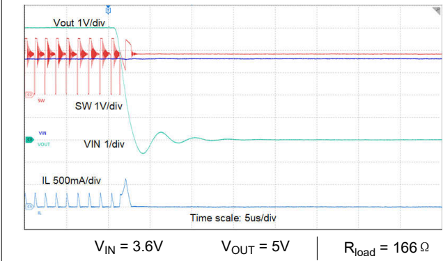
图 8-26. 短路保护
