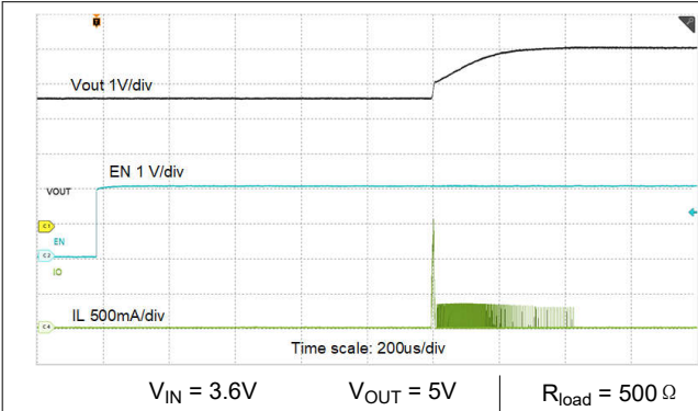
图 8-24. 由 EN 启动
