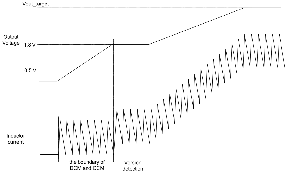
图 7-3. 软启动时序
