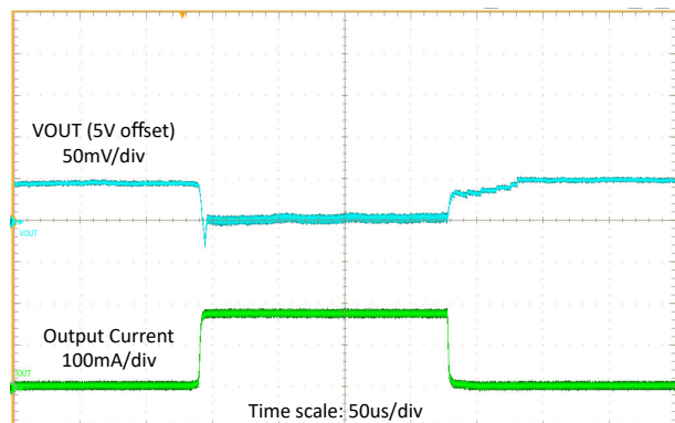
图 8-8. 负载瞬态
