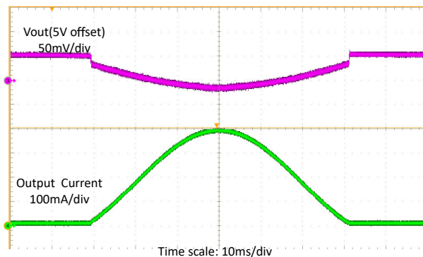
图 8-9. 负载扫描
