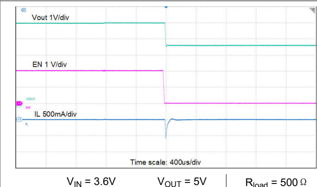
图 8-25. 由 EN 关断
