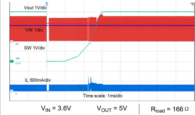
图 8-27. 短路恢复
