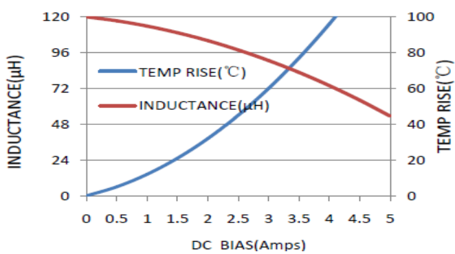
FSA1360-121MT
