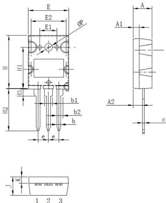
外形名称: TO-264
