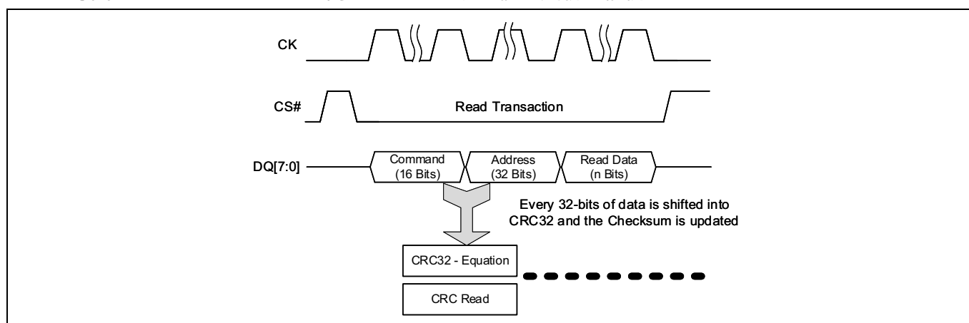
Figure 40 CRC による読み出し保護
