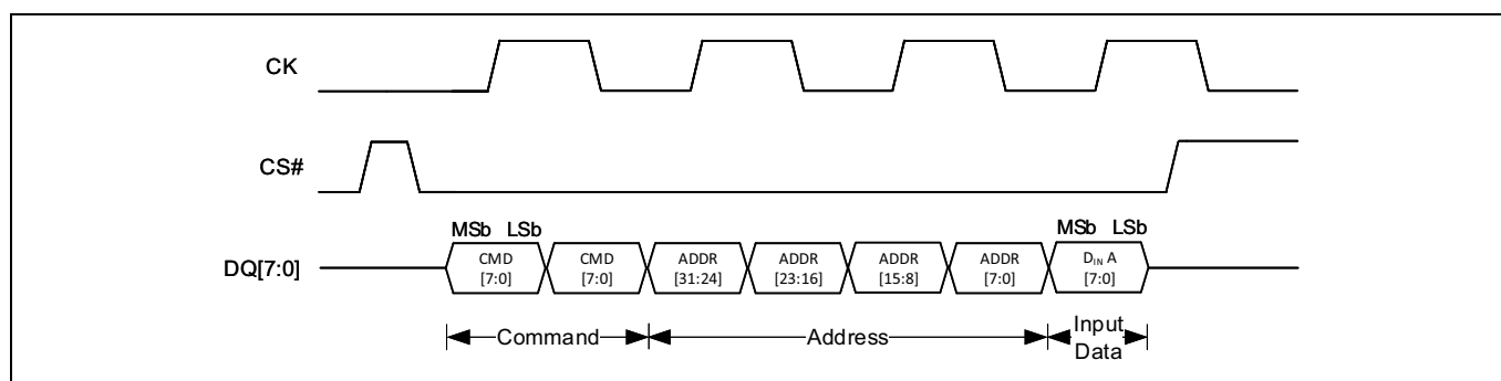
Figure 26 コマンド、アドレスおよびシングル バイト データ入力のあるオクタル DDR プログラム トランザクション [3]
