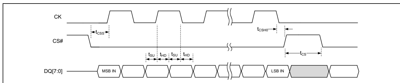
Figure 80 オクタル DDR 入力タイミング
