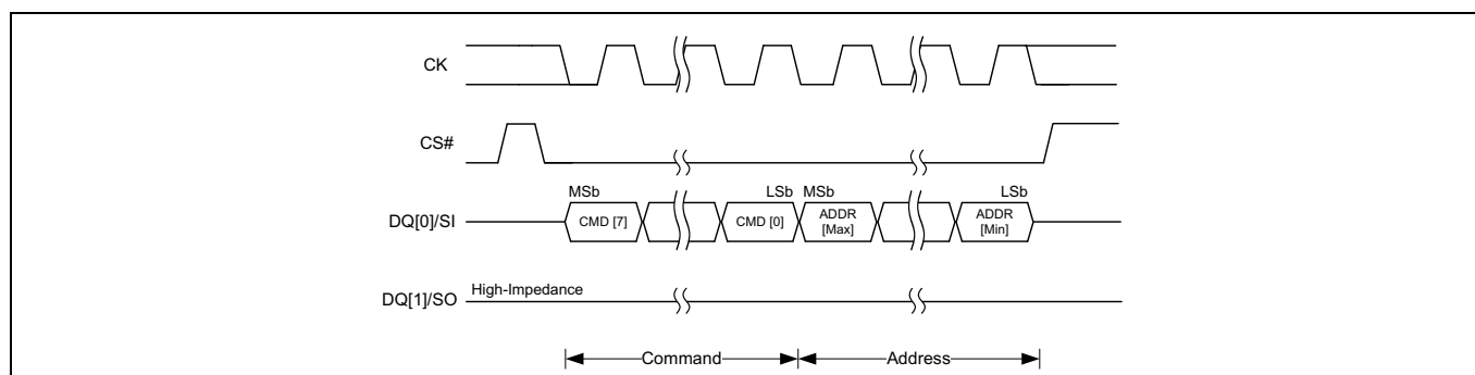
Figure 7 コマンド入力のある SPI トランザクション
