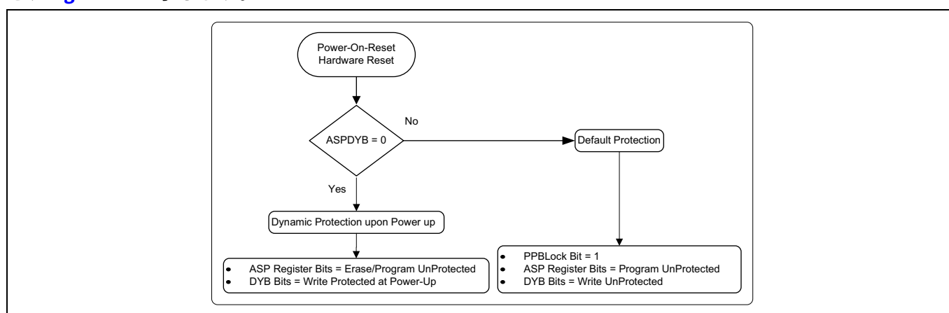
Figure 48 ダイナミック セクタ保護スキームのフローチャート
