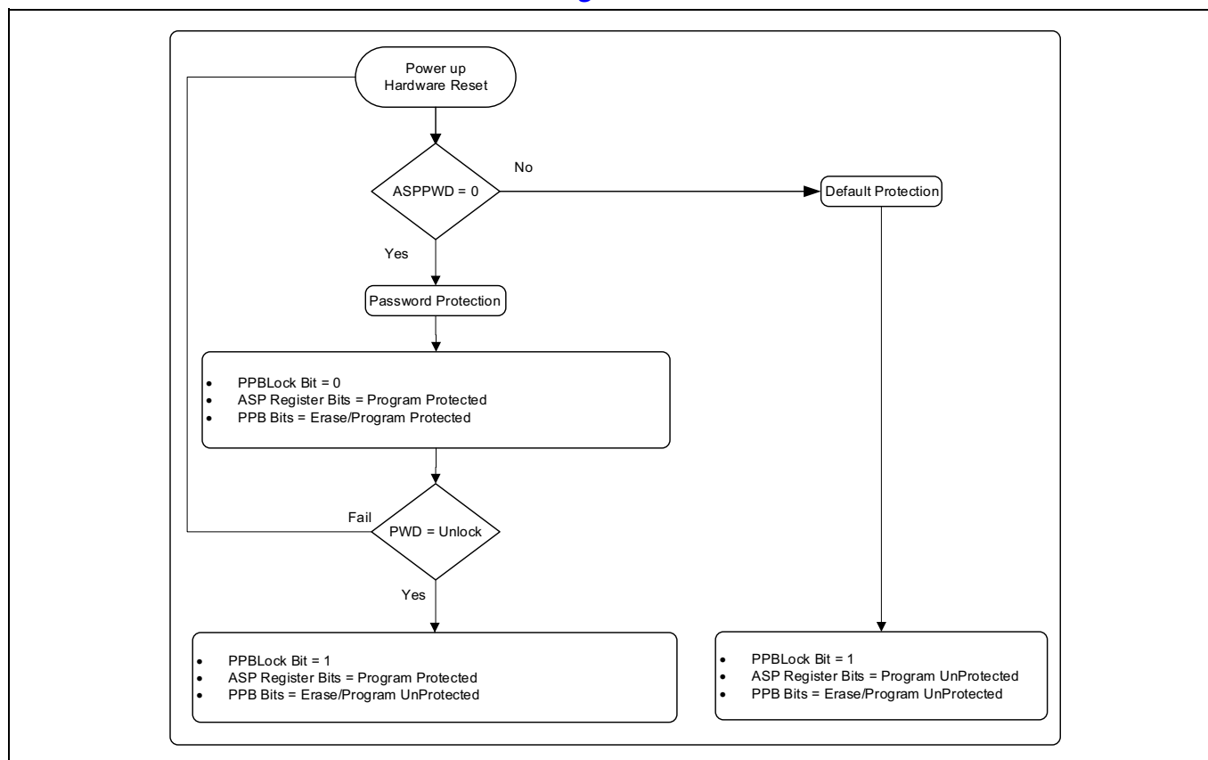
Figure 50 パスワード保護スキームのフローチャート
