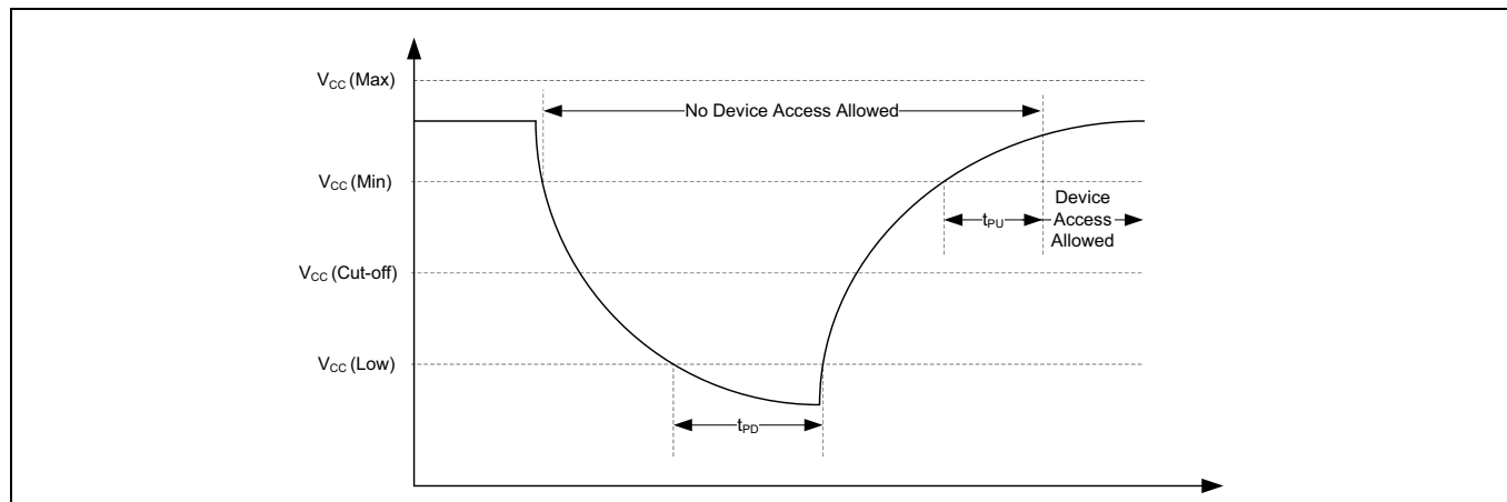
Figure 65 電源切断と電圧低下
