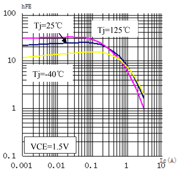
hFE-Ic
