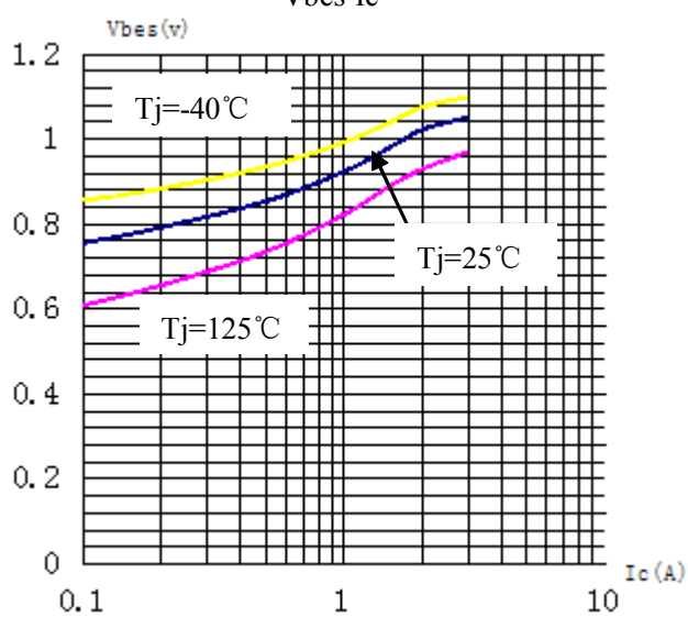
Vbes-Ic
