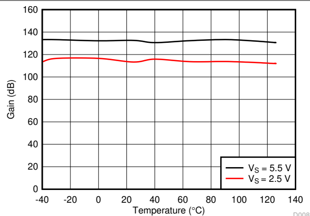
图 5-3. 开环增益与温度间的关系
