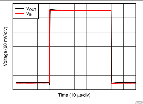
图 5-22. 无相位反转
