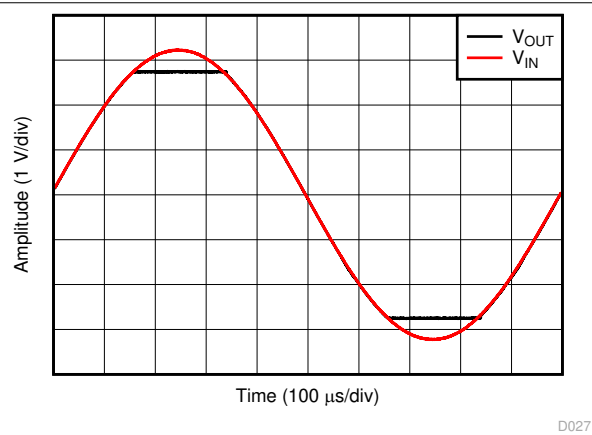
图 5-22. 无相位反转
