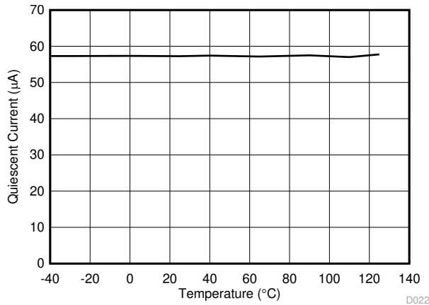
图 5-17. 静态电流与温度间的关系
