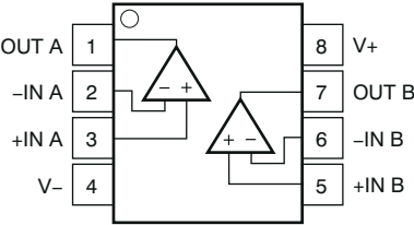
图 4-3. LMV358A D、DDF、DGK 或 PW 封装，8 引脚 SOIC、SOT-23、VSSOP 或 TSSOP (顶视图)
