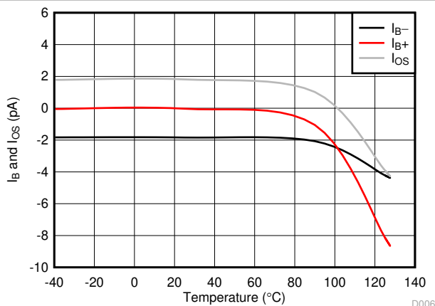
图 5-1. I_B 和 I_{OS} 与温度间的关系
