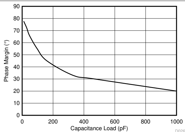
图 5-21. 相位裕度与容性负载间的关系
