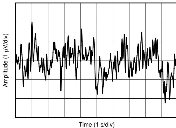
图 5-12. 0.1Hz 至 10Hz 集成电压噪声
