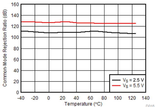
图 5-11. 直流 CMRR 与温度间的关系
