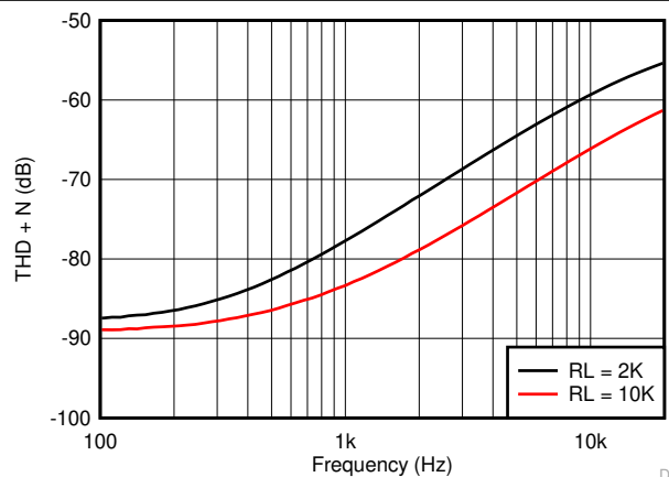
图 5-14. THD+N 与频率间的关系
