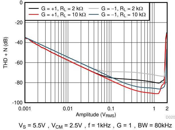
图 5-15. THD + N 与幅度间的关系
