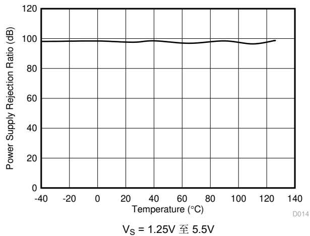
图 5-9. 直流 PSRR 与温度间的关系
