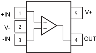
图 4-2. LMV321AU DBV、LMV321A DCK 封装 5 引脚 SOT-23、SC70 顶视图
