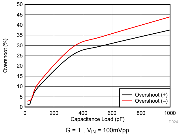
图 5-19. 小信号过冲与容性负载间的关系
