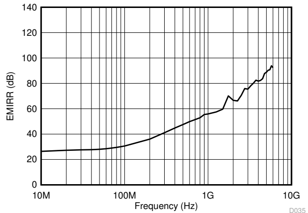
图 5-30. 以同相输入为基准的电磁干扰抑制比 (EMIRR+) 与频率间的关系
