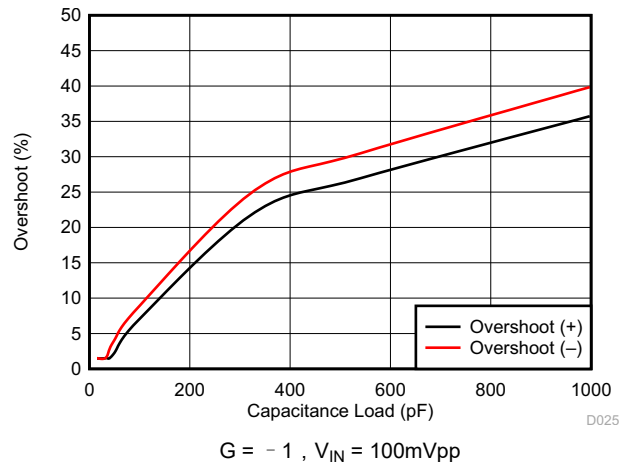
图 5-20. 小信号过冲与容性负载间的关系
