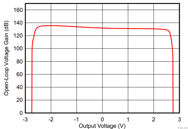
图 5-5. 开环增益与输出电压间的关系
