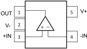
图 4-1. LMV321A DBV 封装 5 引脚 SOT-23 顶视图
