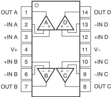
图 4-4. LMV324A D、DYY、PW 封装，14 引脚 SOIC、SOT-23、TSSOP（顶视图）
