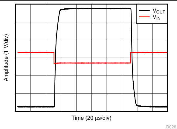
图 5-23. 过载恢复
