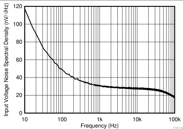
图 5-13. 输入电压噪声频谱密度
