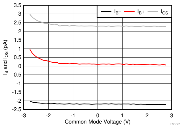
图 5-2. I_B 和 I_{OS} 与共模电压间的关系
