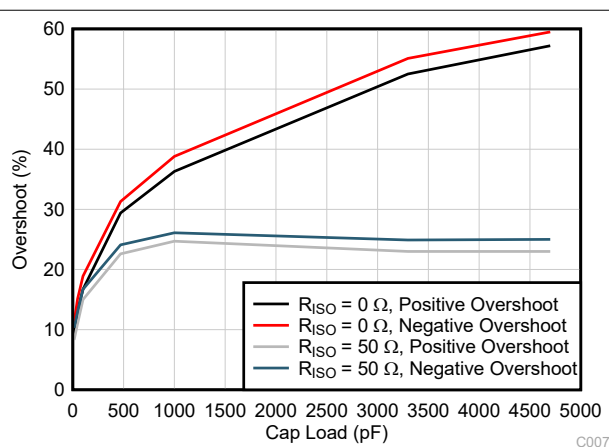
图 7-6. 小信号过冲与容性负载之间的关系 (10mV 输出阶跃, G = -1 )
