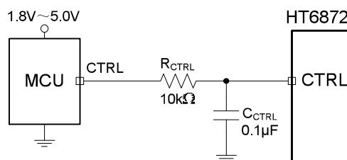
图2 微控制器单端控制CTRL
