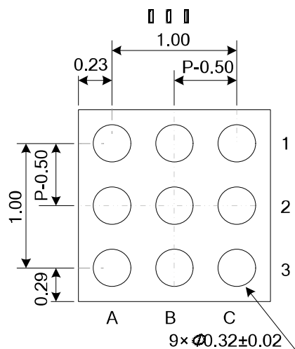
9焊球WLCSP
