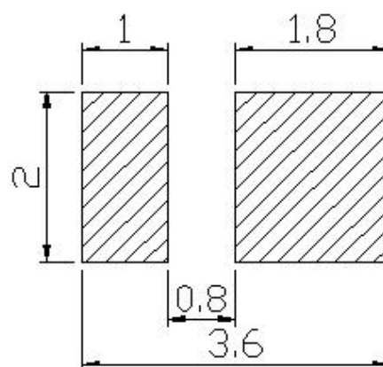
焊盘建议图
