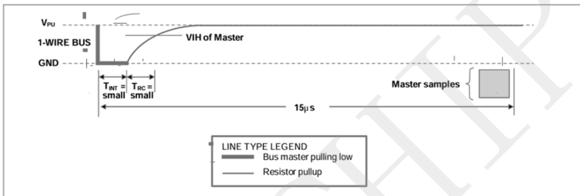
图 19.推荐的控制度 1 时序
