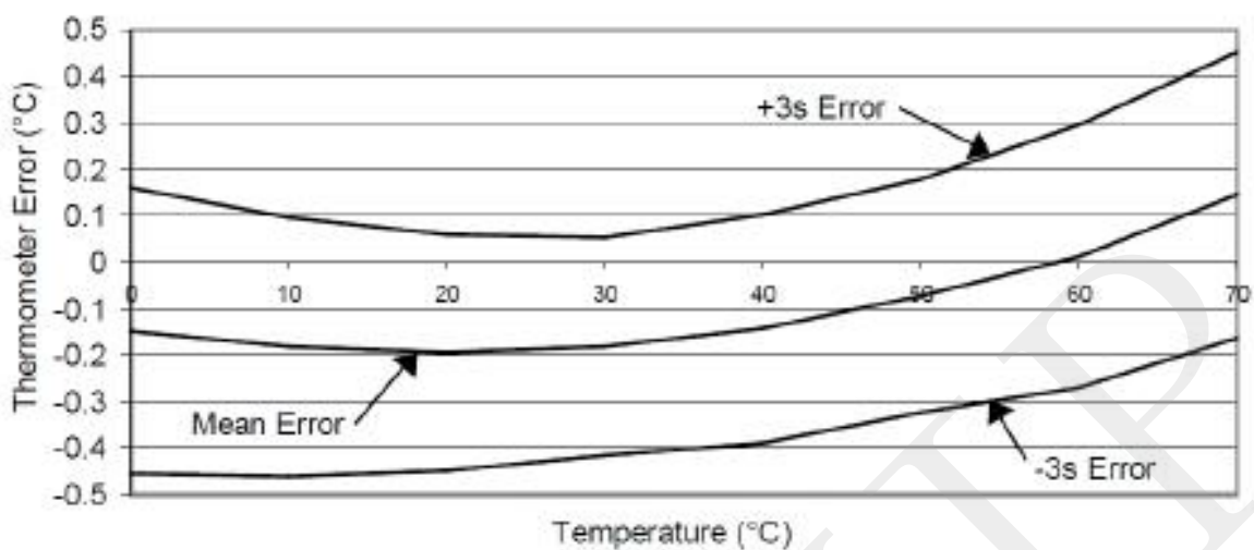
图 3.典型特性曲线
