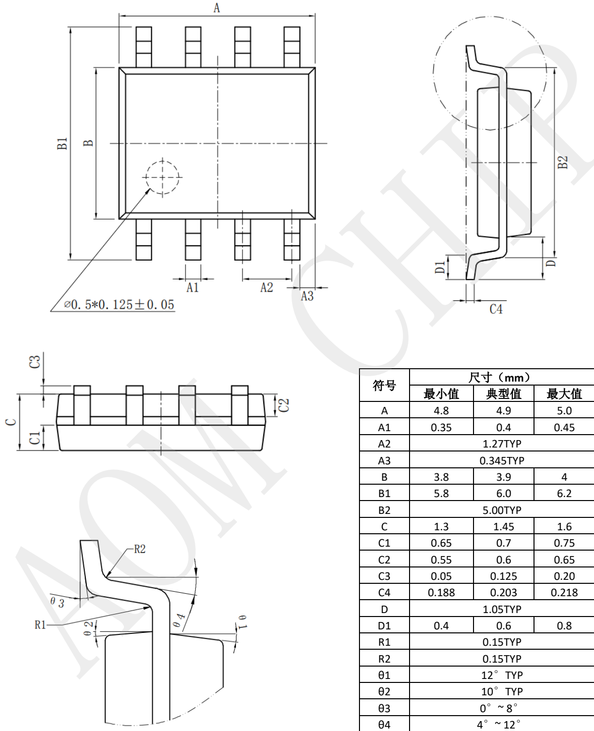
图 20.SOP8 封装尺寸图
