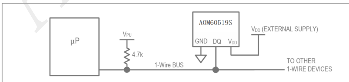
图 8. 使用外部电源为 AOM60519S 供电
