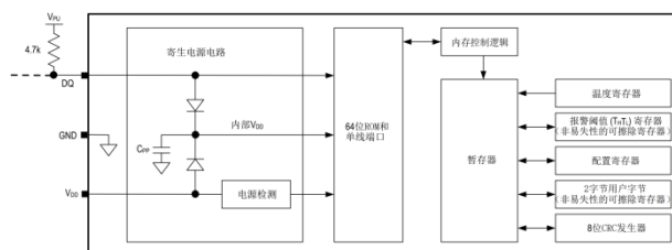
图 1. 典型应用框图
