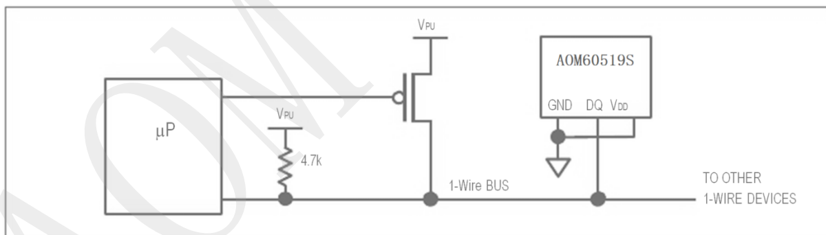
图 7. 在温度转换期间为寄生供电的 AOM60519S 供电
