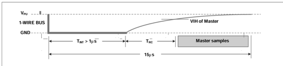
图 18.控制器读 1 的详细时序
