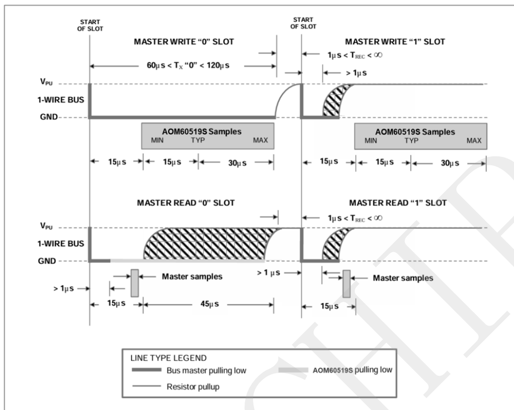
图 17.读/写时序图
