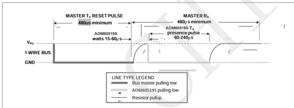
图 16. 初始化时序
