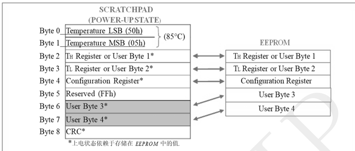
图 10. AOM60519S 内存映射
