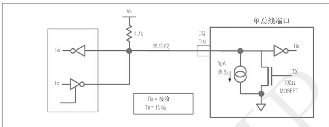
图 13. 硬件结构图
