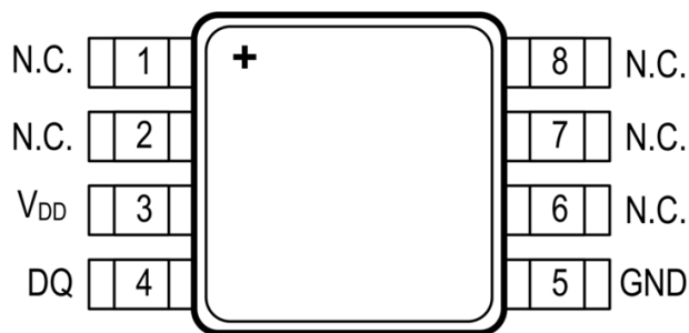
图 2.SOP8 脚位图（顶视图）
