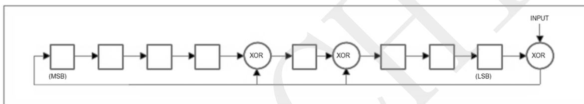
图 12.CRC 产生器
