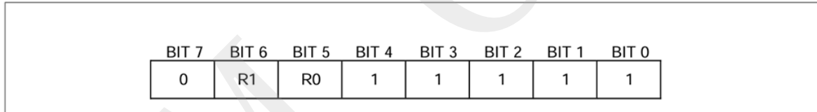
图 11.配置寄存器
