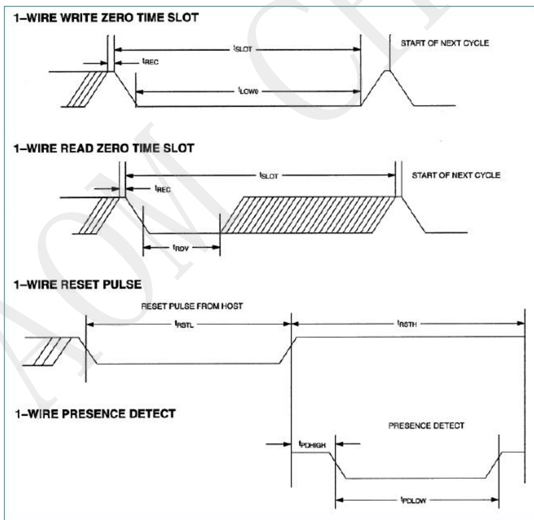
图 4.时序图
