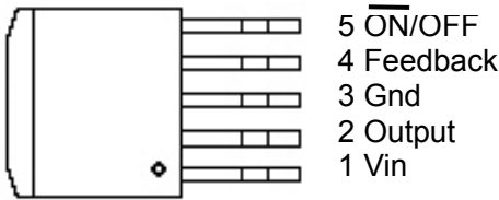
TO263-5L
