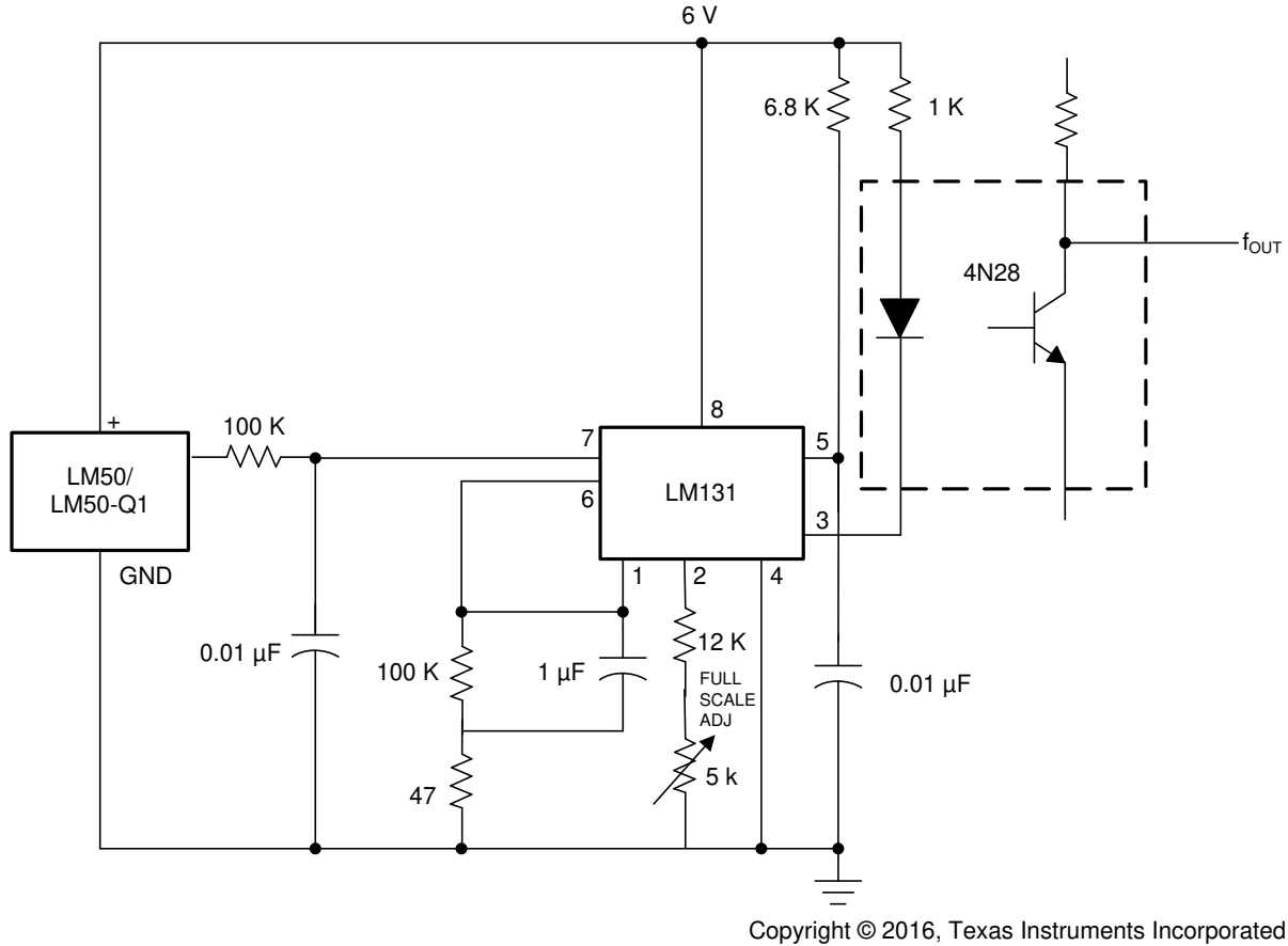
图 8-7. 具有压频转换器和隔离式输出的 LM50-Q1
