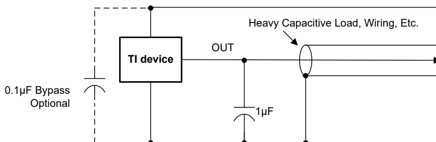
图 8-3. 适用于嘈杂环境带滤波器的 LM50-Q1
