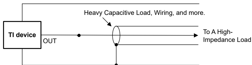
图 8-2. LM50-Q1 容性负载无需去耦
