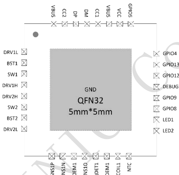
图 1 IP6802 引脚图
