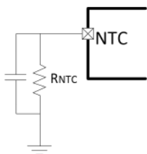
图 6 NTC 检测电路
