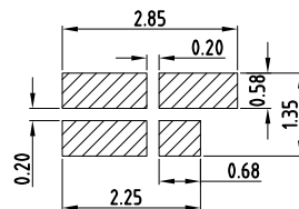
METAL MASK T=0.10 TOLERANCE±0.05(钢网推荐图)
