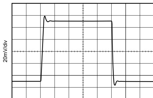
图 15. 小信号阶跃响应
