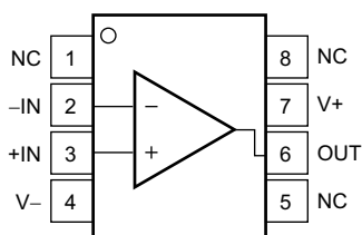
OPA348 D 封装 8 引脚 SOP 俯视图
