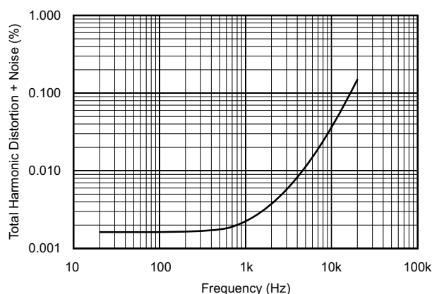
图 18. 总谐波失真 + 噪声与频率间的关系
