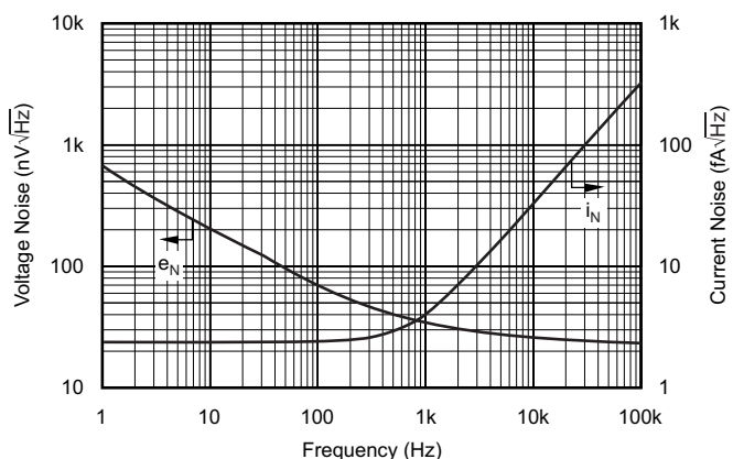
图 17. 输入电流和电压噪声频谱密度与频率间的关系
