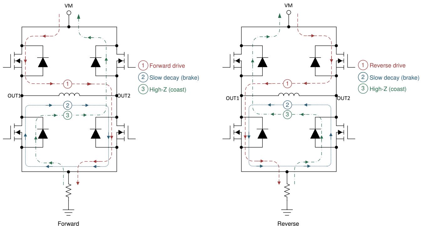
图 7-1. H 桥状态
