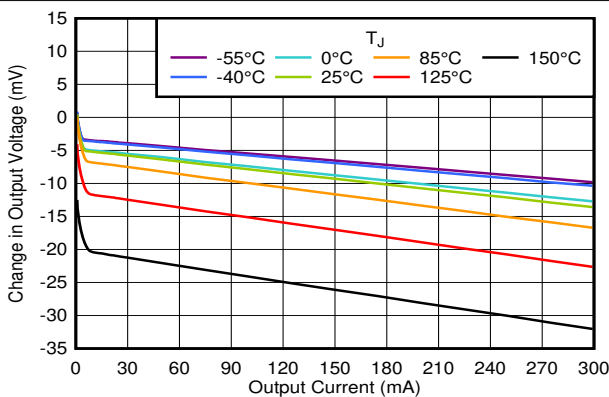
图 5-7. Load Regulation vs I_{OUT}
