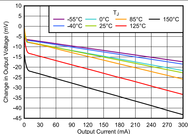
图 5-9. Load Regulation vs I_{OUT}
