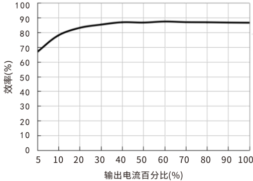
效率Vs输出负载(Vin=5V) VRB0524ZP-6WR3
