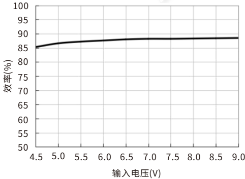
效率Vs输入电压(满载) VRB0524ZP-6WR3
