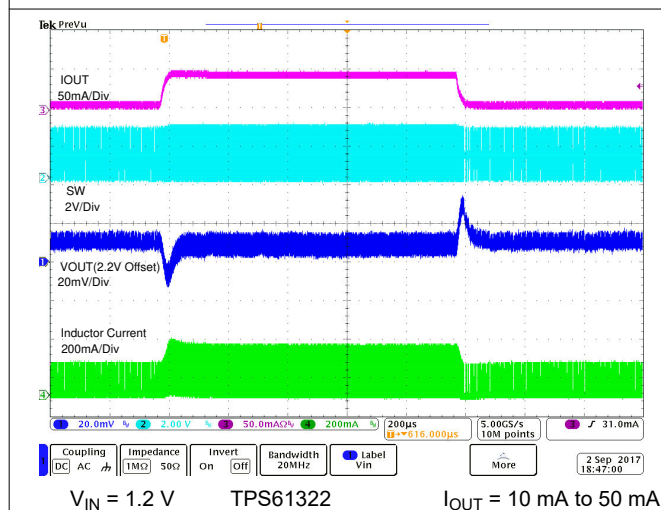
图 8-6. Load Transient
