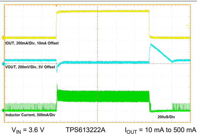
图 8-16. Load Transient
