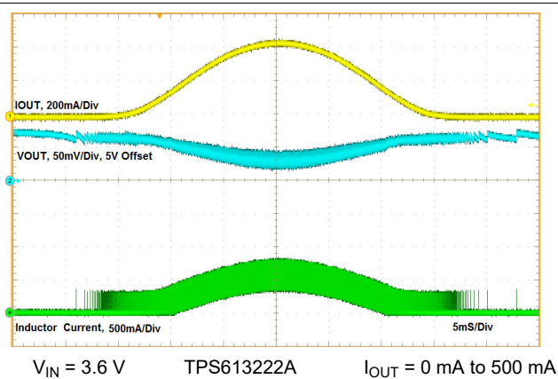
图 8-17. Load Regulation
