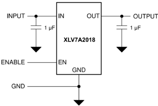
电路连接图
