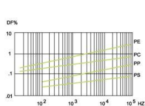
损耗角正切与频率的关系 Dissipation Factor vs. Frequency
