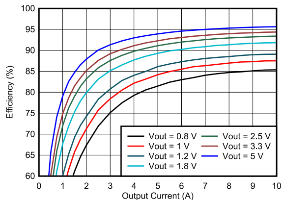
图 6-4. TPS546A24A 效率与输出电流间的关系
