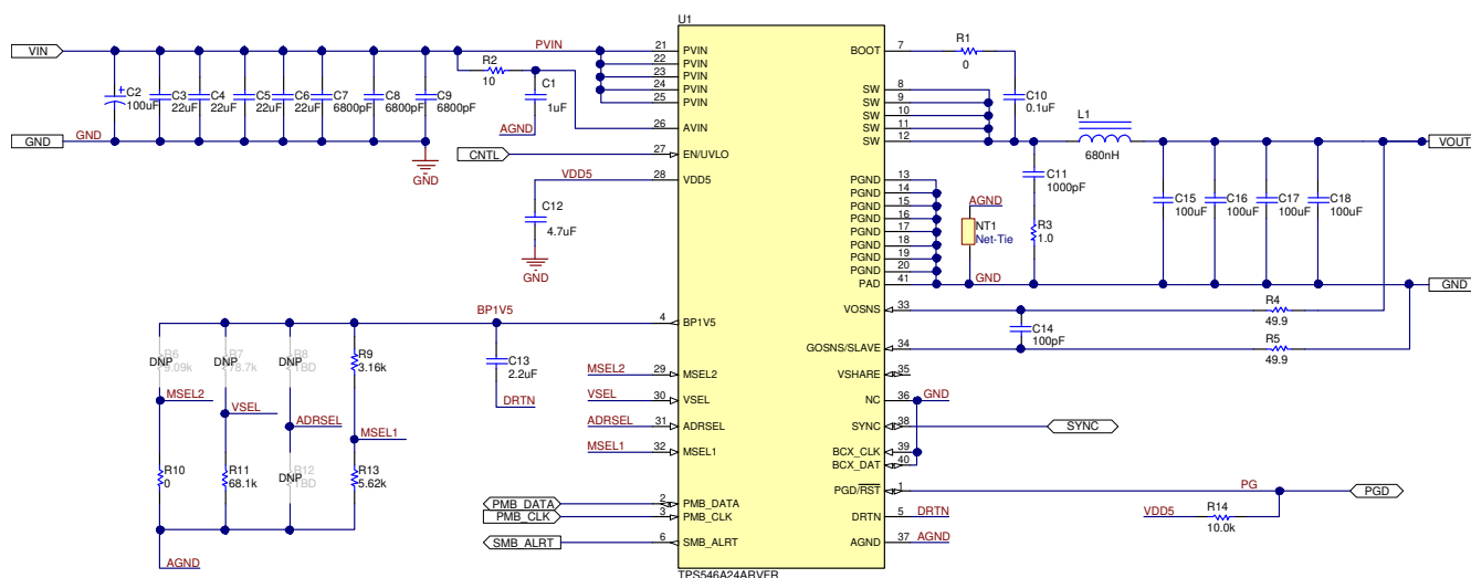
图 8-1. TPS546A24A 应用
