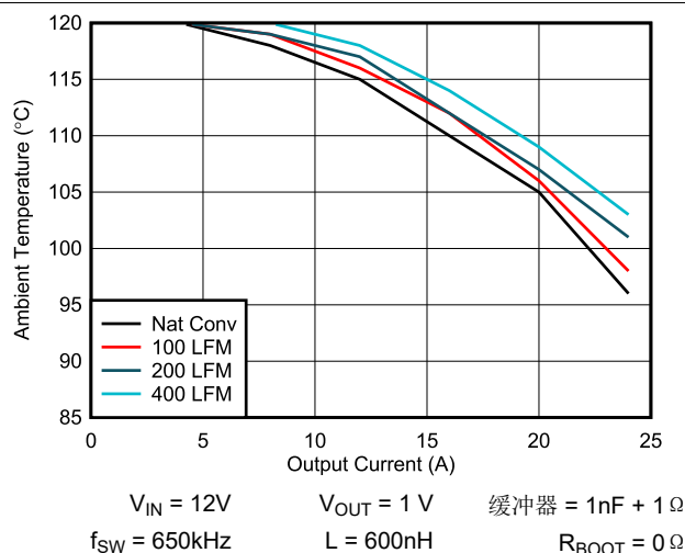
图 6-1. TPS546A24A 安全工作区
