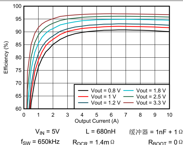
图 6-2. TPS546A24A 效率与输出电流间的关系
