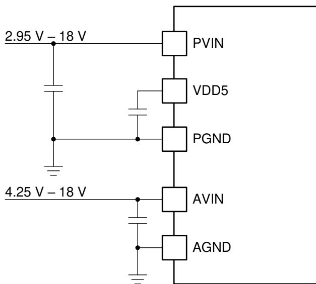
图 7-2. TPS546A24A 单独的 PVIN 和 AVIN 连接
