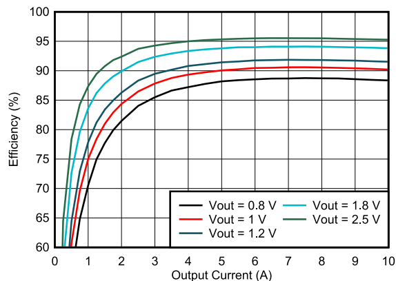
图 6-3. TPS546A24A 效率与输出电流间的关系
