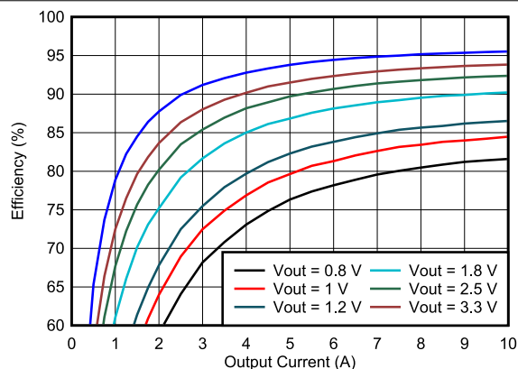
图 6-5. TPS546A24A 效率与输出电流间的关系
