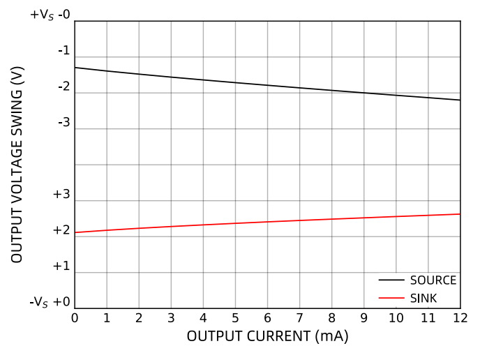
图 12 输出电压摆幅随输出电流的变化 ( G = 1 )
