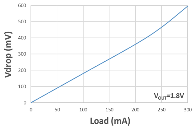
Fig 11. V_{DROP} vs 负载
