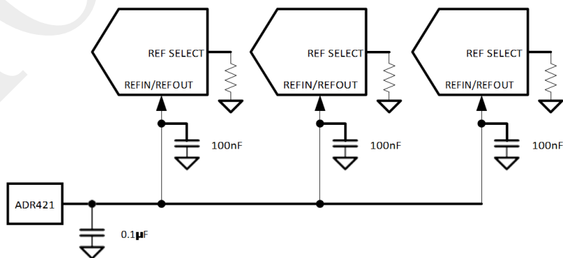
图 34. 一个外部基准电压源驱动多个 AOM67484 REFIN 引脚
