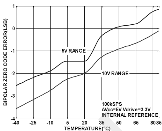
图 17. 双极性零代码误差与温度的关系
