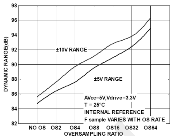
图 23.动态范围与过采样倍率的关系
