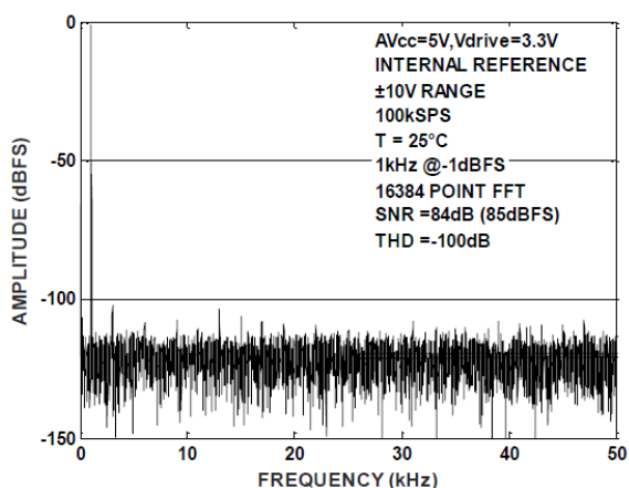
图 9. AOM67484 FFT±10V 范围
