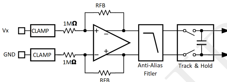
图 28.模拟输入电路
