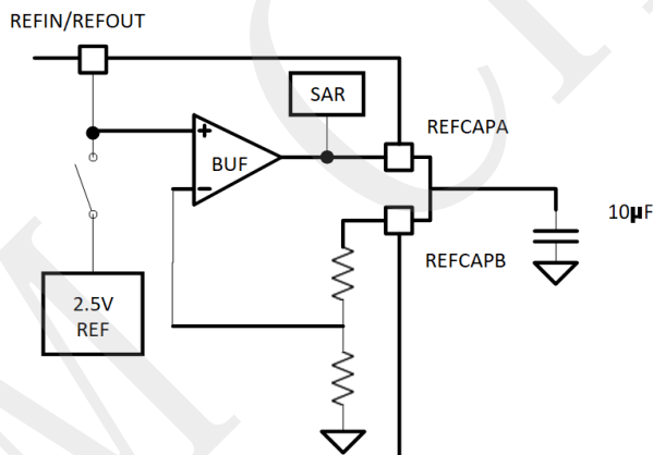
图 33. 基准电压电路
