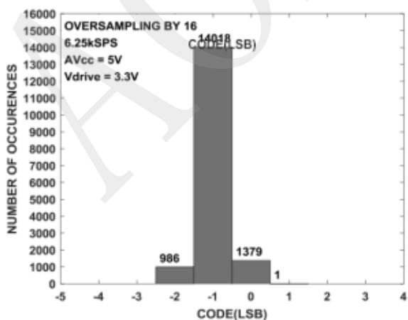
图 46. 码直方图：16 倍过采样
