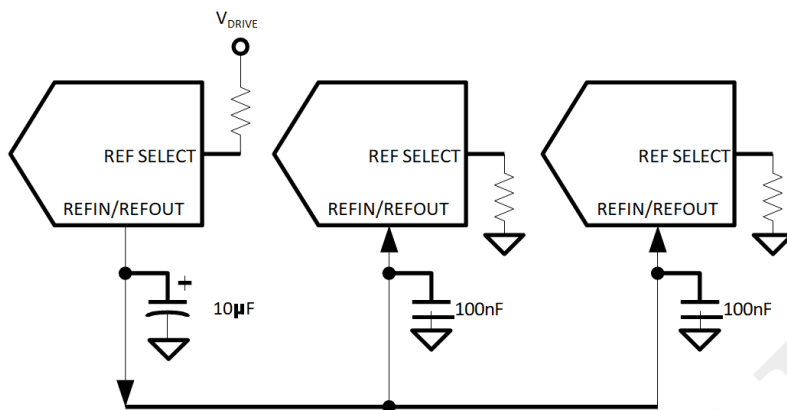
图 35.内部基准电压源驱动多个 AOM67484 REFIN 引脚
