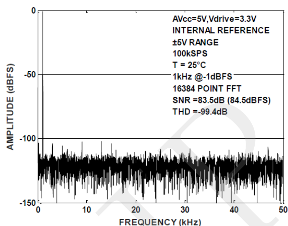
图 10. AOM67484 FFT±5V 范围
