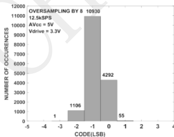
图 45. 码直方图：8 倍过采样
