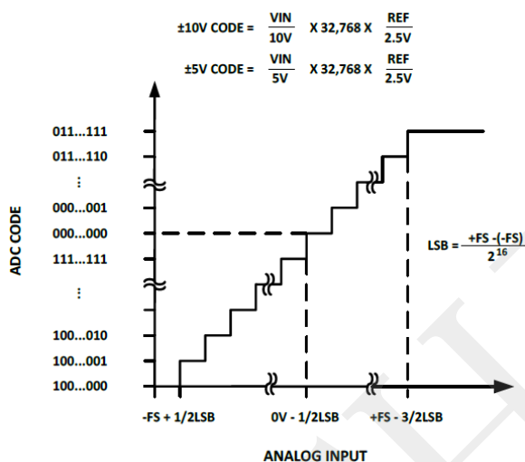
图 32.AOM67484 传递特性
