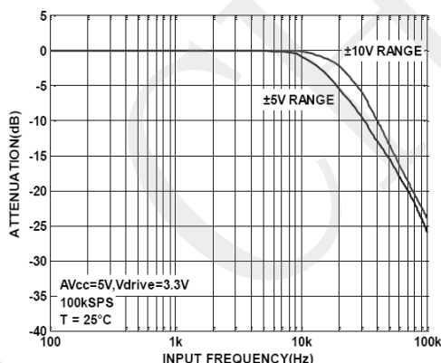
图 31. 模拟抗混叠滤波器频率响应
