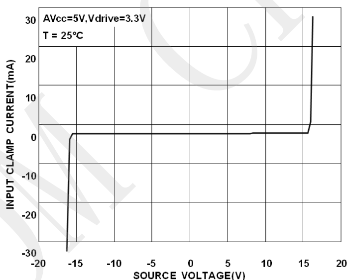
图 29.输入箝位保护特性
