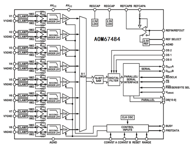
图 1.功能框图
