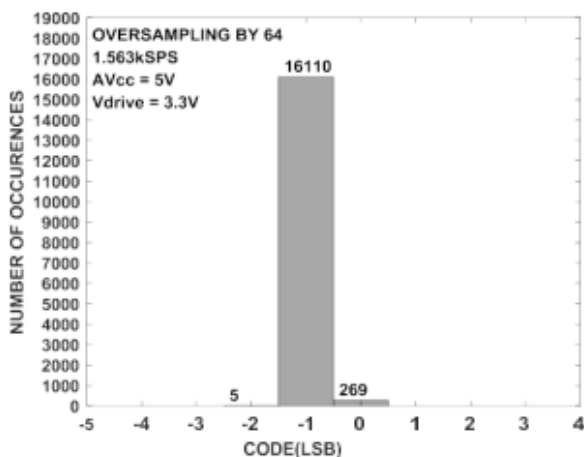
图 48.码直方图：64 倍过采样
