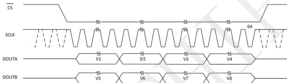
图 39.采用双 DOUT 线路的 AOM67484 串行接口
