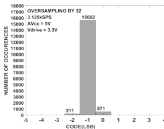
图 47. 码直方图：32 倍过采样
