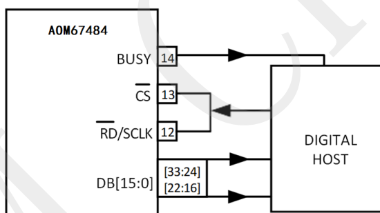
图 38. 一个 AOM67484 使用并行总线-和短接在一起
