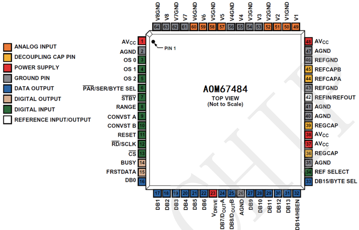
图 8. AOM67484 引脚配置（顶视图）
