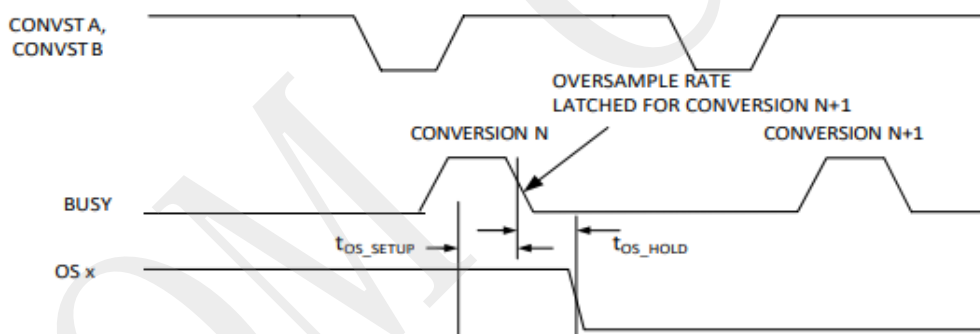
图 41. OSx 引脚时序
