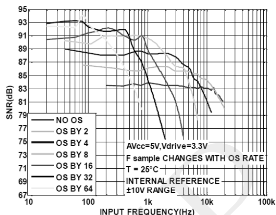
图 22.不同过采样倍率下 SNR 与输入频率的关系, \pm 10V 范围图
