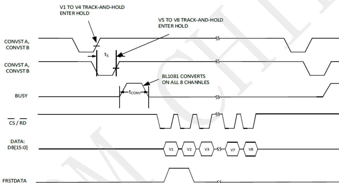
图 37.AOM67484 分两组通道同步采样，使用独立的 CONVSTA 和 CONVSTB-并行模式
