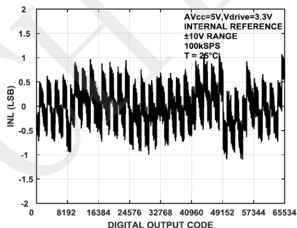
图 12. AOM67484 典型 INL, ±10V 范围
