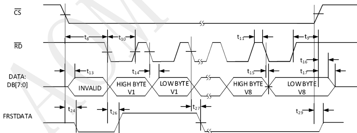
图 7. 字节模式读取操作
