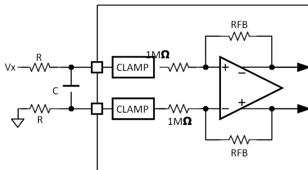
图 30. AOM67484 模拟输入端上的输入电阻匹配
