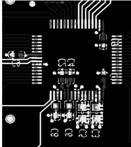
图 49.AOM67484 外围去耦
