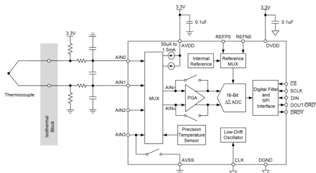
图 1.AOM67008 功能框图
