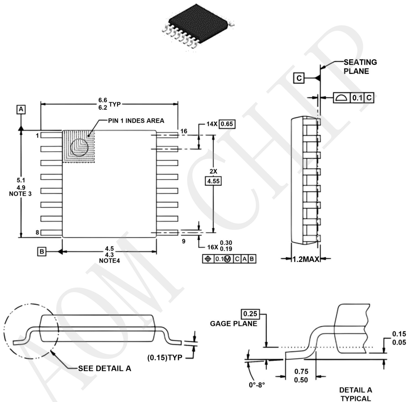
图 3. 封装尺寸图
