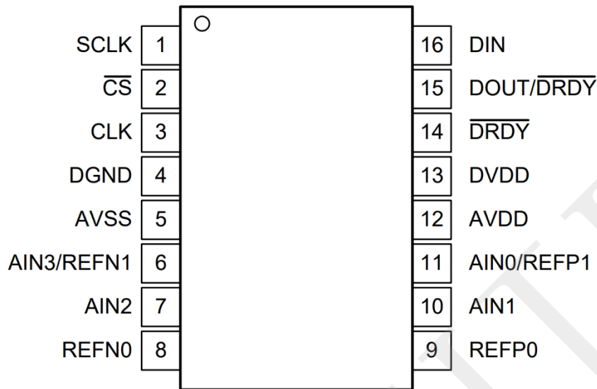
图 2.AOM67008 引脚框图（顶视图）
