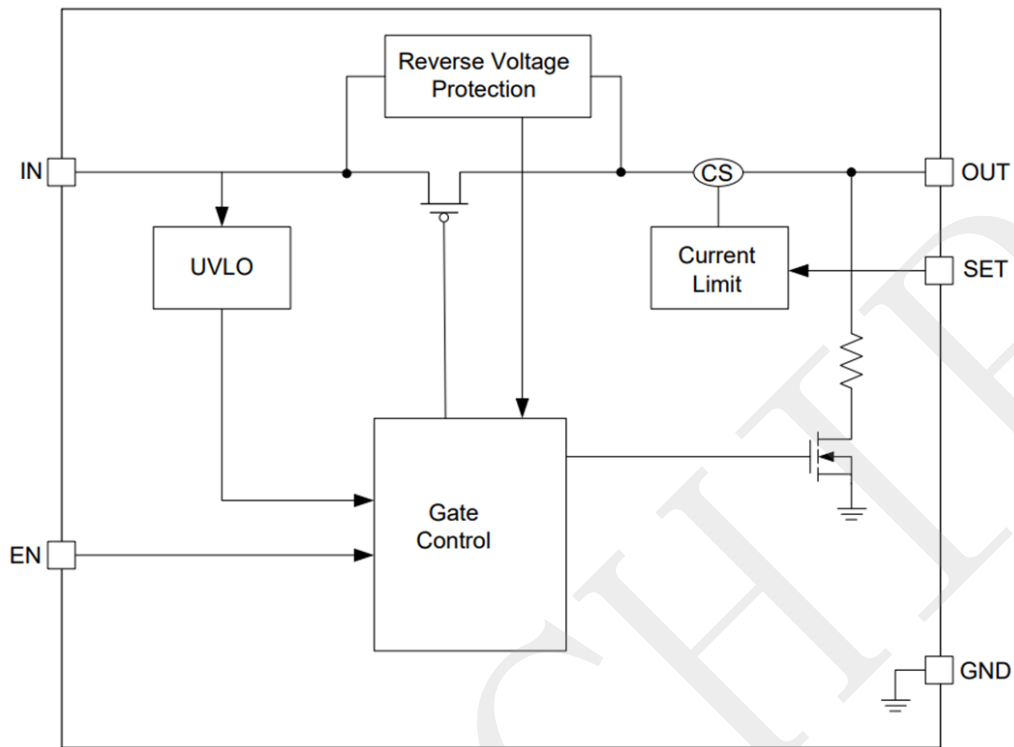
图 2. AOM64873T 基本框图
