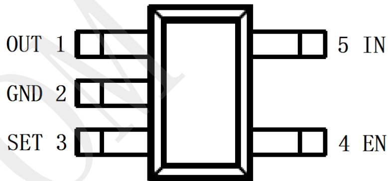
图 3. SOT23-5L 封装脚位图
