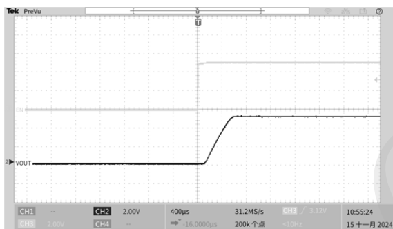
图 6. EN 启动 (EN=5V, PWM), VIN= 5V, RL=20Ω
