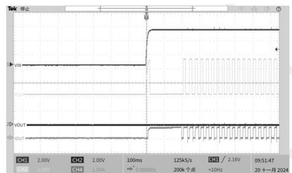
图 10. 输出短路上电响应 VIN=5V, VEN=5V
