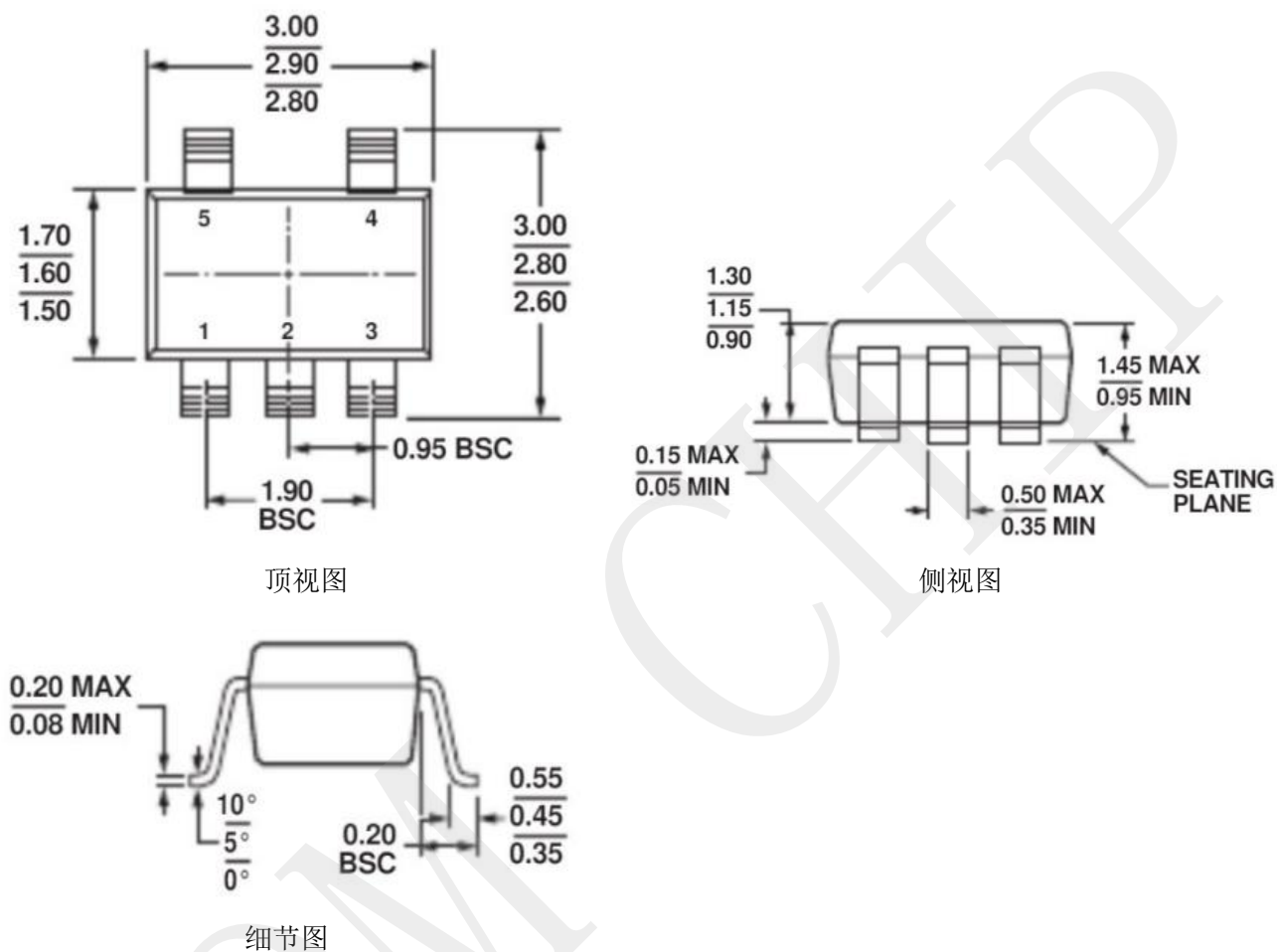
图 12. SOT23-5L 封装尺寸图
