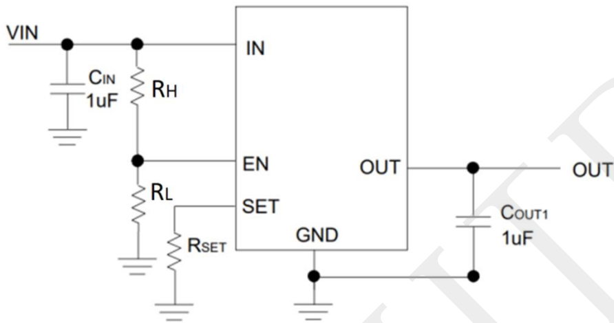
图 11.AOM64873T 典型应用推荐电路
