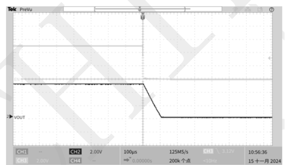
图 7. EN 关断 (EN=5V, PWM), VIN= 5V, RL=20Ω
