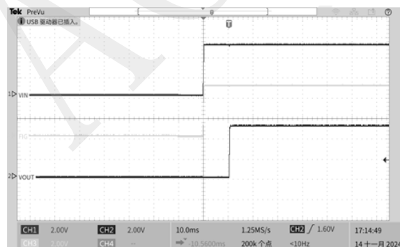
图 9. 输出延时 VIN=VEN=5V, RL=20K
