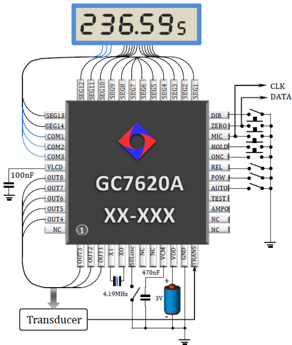
GC7620A 应用电路
