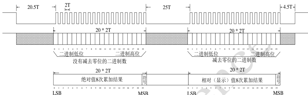
7620A 串口同步时钟和数据信号波形图
