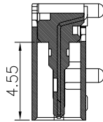
剖面图 A-A
