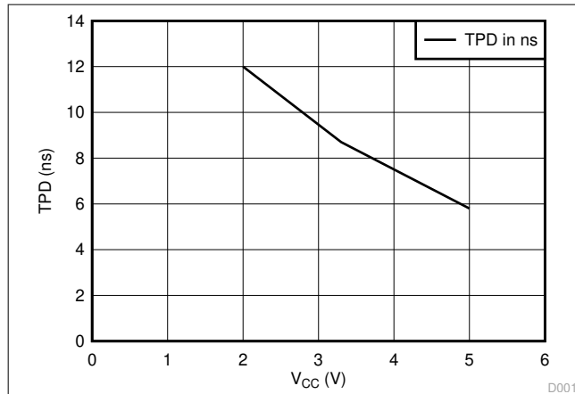
图 5-1. TPD 与 V CC 间的关系
