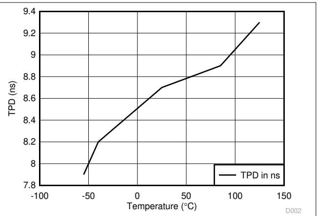
图 5-2. TPD 与温度间的关系
