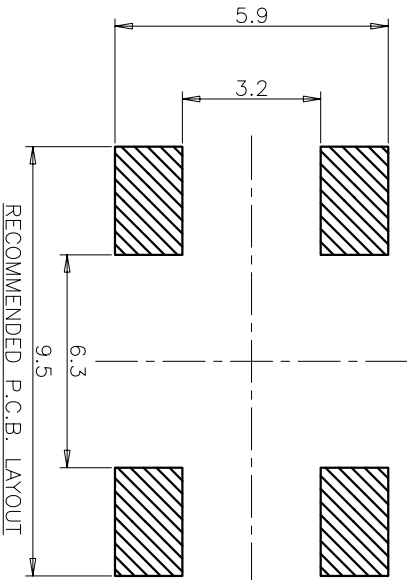
安装尺寸图 RECOMMENDED P.C.B. LAYOUT
