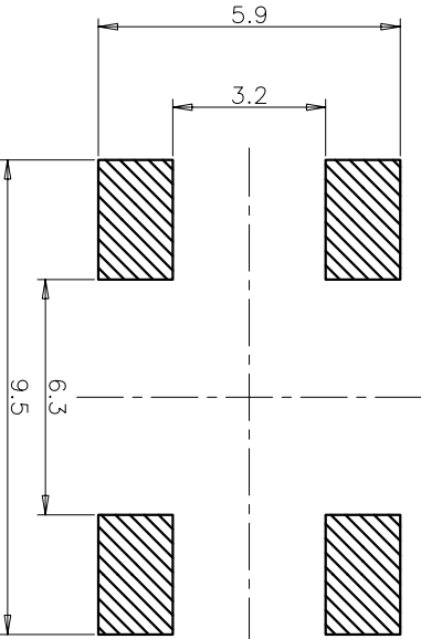
安装尺寸图
