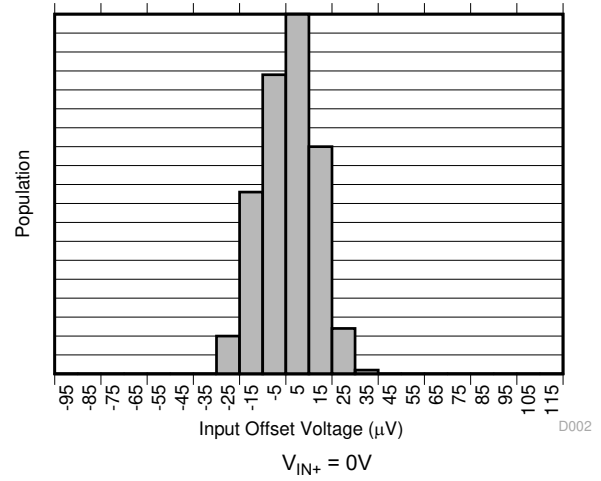
图 7-2. 输入失调电压产生分布图 A2
