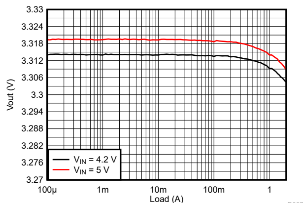
图 9-101. Load Regulation
