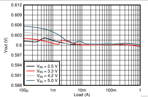
图 9-16. Load Regulation
