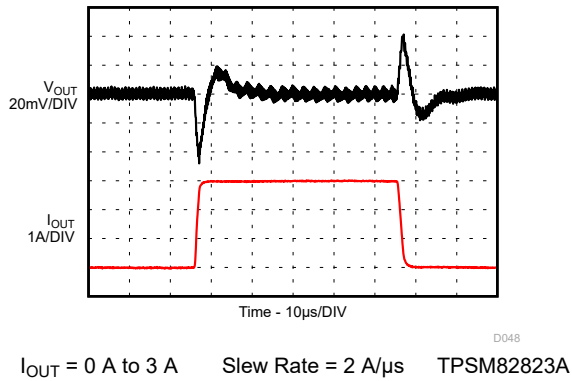
图 9-157. Load Transient
