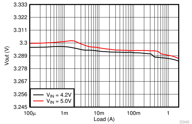
图 9-68. Load Regulation
