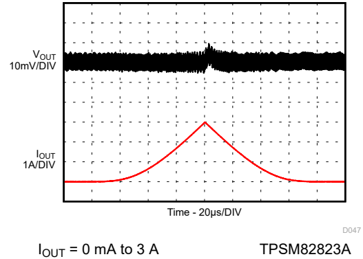
图 9-156. Load Sweep
