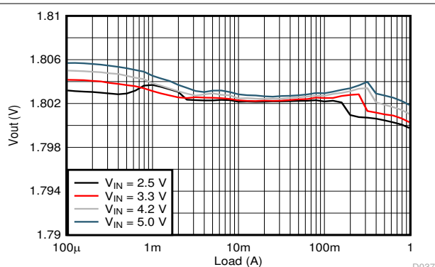
图 9-18. Load Regulation
