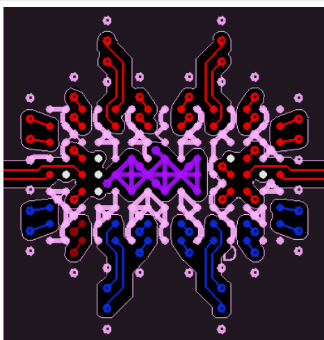
图 7-8. Top Layer
