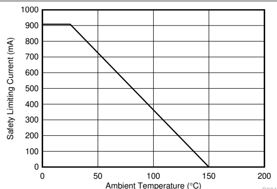
图 6-6. D-8 封装根据 VDE 标准限制功率的热降额曲线
