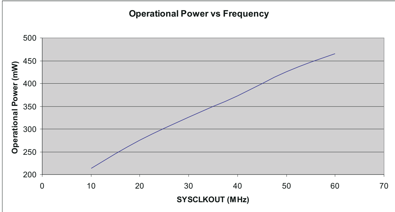
图 6-2. 典型运行功率与频率间的关系 (F2803x)
