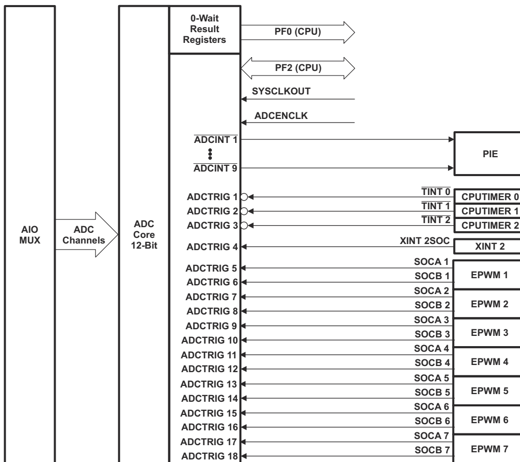
图 7-17. ADC 连接
