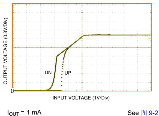
图 7-5. UVLO Thresholds
