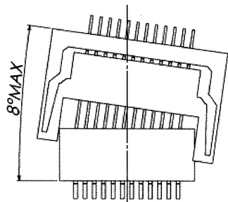
図1/Fig. 1(水平接続タイプに適用/ Apply to horizontal connection)
