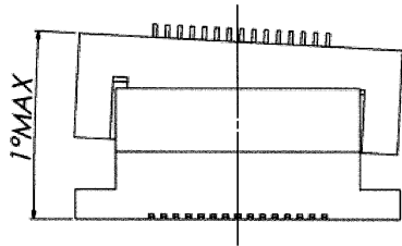
図3/ Fig.3(垂直接続タイプに適用/ Apply to vertical connection)
