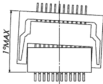
図3/ Fig. 3(水平接続タイプに適用/ Apply to horizontal connection)
