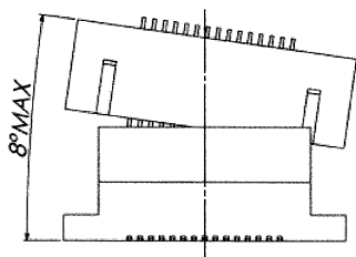
図1/Fig.1(垂直接続タイプに適用/Apply to vertical connection)
