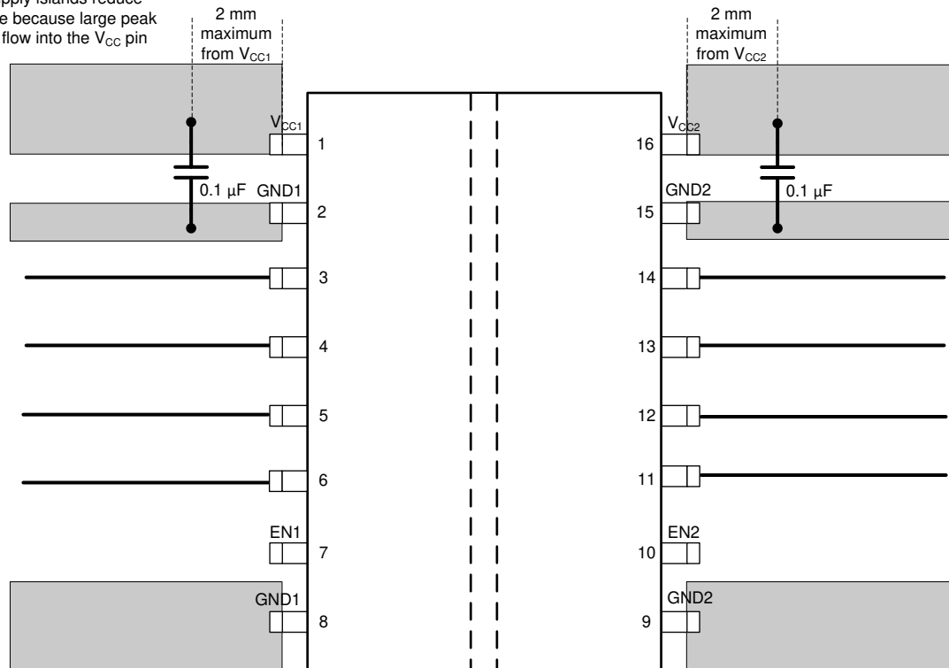
图 8-9. 布局示例
