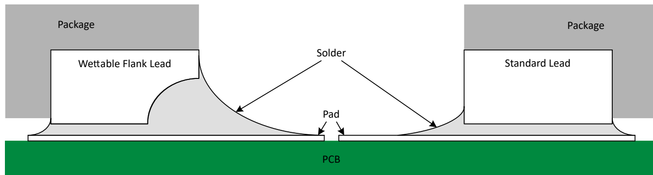
图 9-3. 焊接后具有可润湿侧翼的 QFN 封装和标准 QFN 封装的简化剖面图
