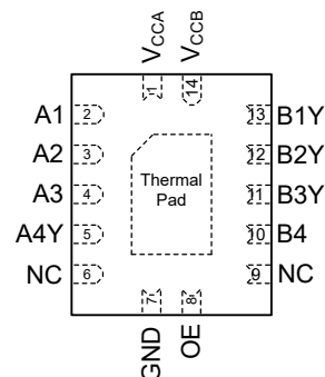
图 6-2. WBQA 封装，14 引脚 VQFN 透明 (顶视图)
