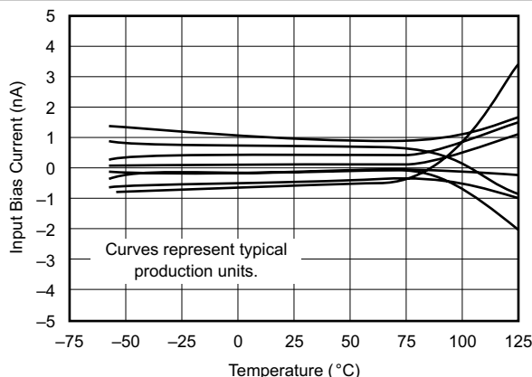
图 7-6. OPA2277 输入偏置电流
