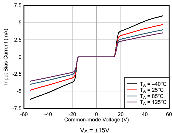
图 7-2. OPAx206 输入电流与输入电压 ( V_S = \pm 15\text{V} ) 间的关系
