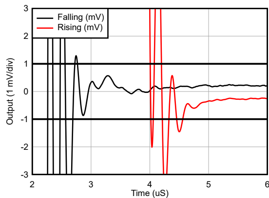
图 5-38. 建立时间
