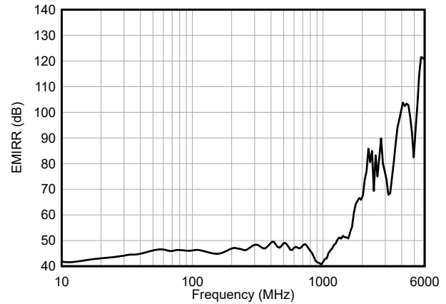
图 5-44. 电磁干扰抑制 (EMIRR)
