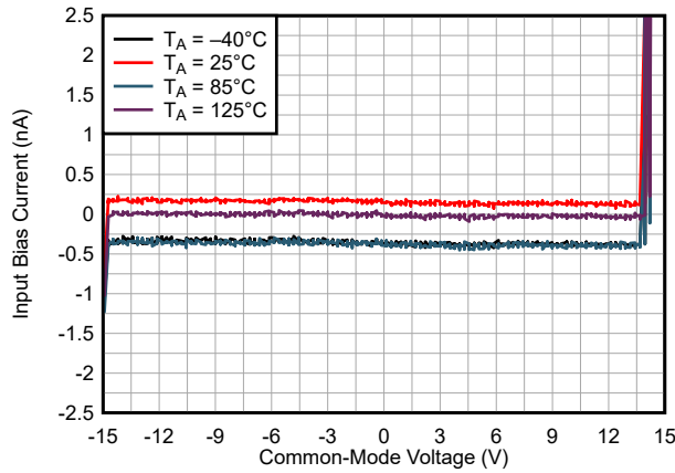
图 5-19. 输入偏置与共模电压间的关系
