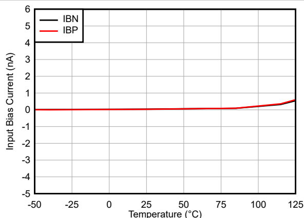
图 7-7. OPAx206 超 \beta 输入偏置电流
