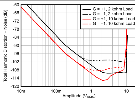
图 5-26. 总谐波失真 + 信噪比与输出振幅间的关系
