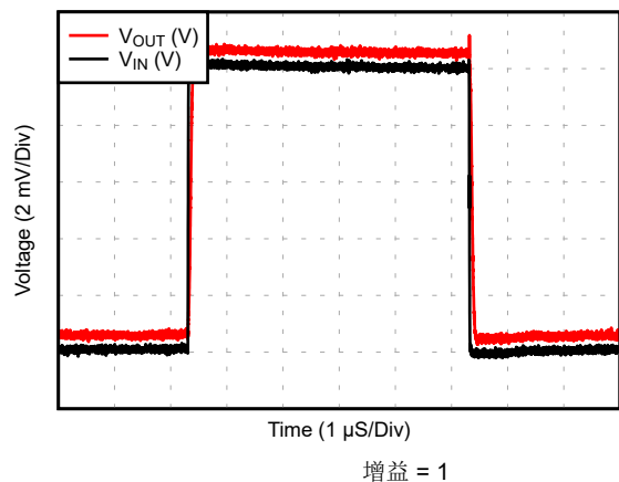
图 5-39. 小信号阶跃响应
