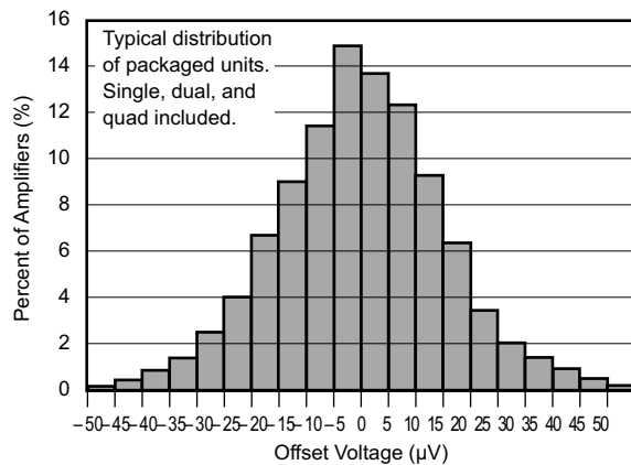
图 7-3. OPA2277 激光微调运算放大器失调电压
