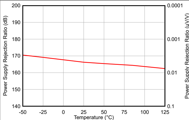
图 5-8. 电源抑制比与温度间的关系
