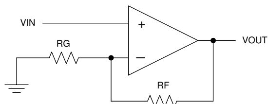
图 8-6. 原理图表示
