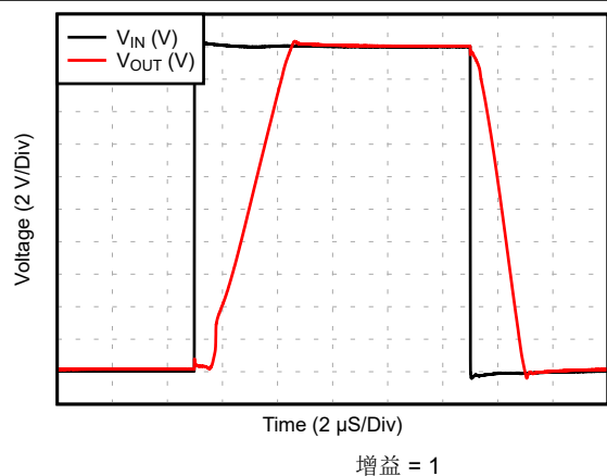
图 5-41. 大信号阶跃响应
