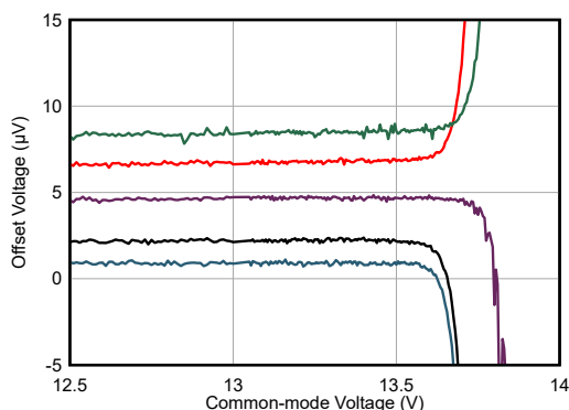
图 5-13. 在高电源电压下失调电压与 V_{CM} 间的关系
