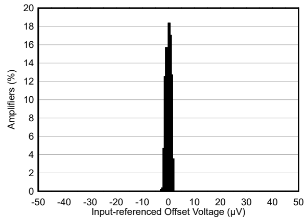
图 7-4. OPAx206 e-trim™ 运算放大器失调电压
