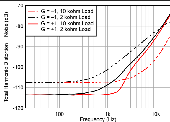
图 5-25. 总谐波失真 + 信噪比与频率间的关系
