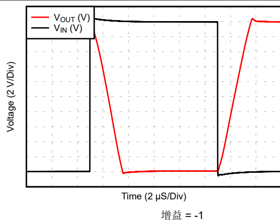
图 5-42. 大信号阶跃响应
