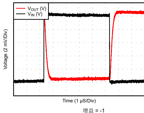
图 5-40. 小信号阶跃响应
