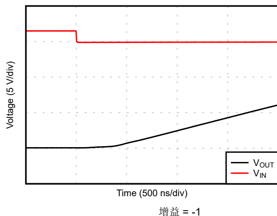
图 5-37. 负过载恢复
