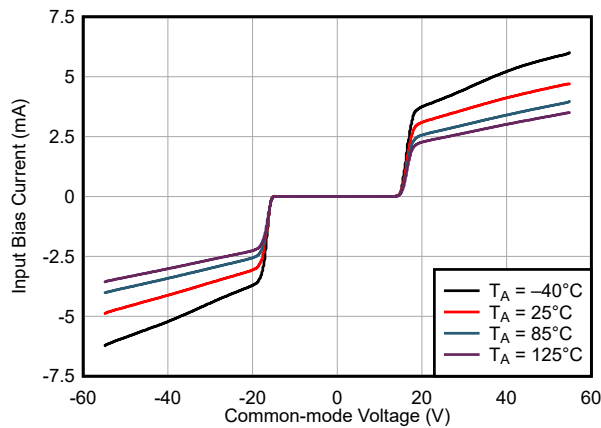
图 5-19. 输入偏置与共模电压间的关系
