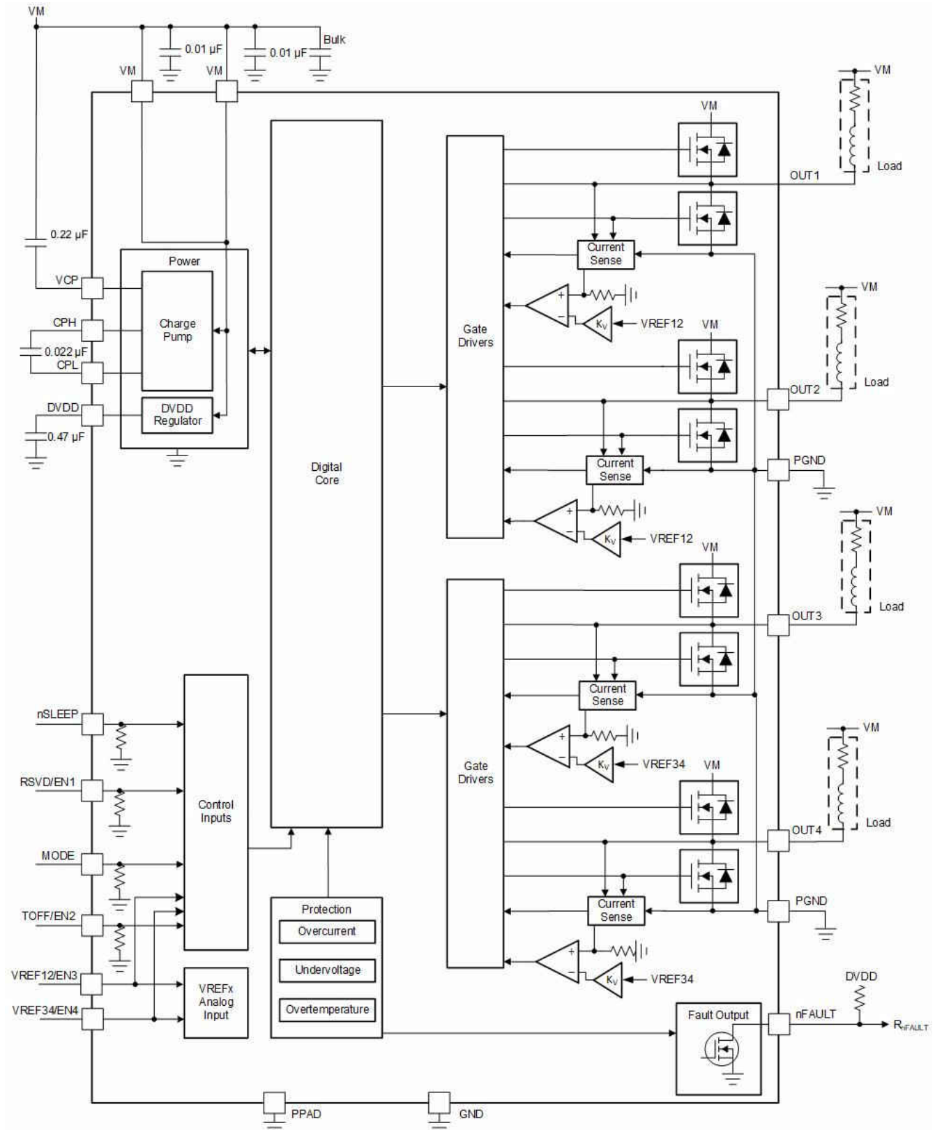
图 7-1. DRV8955 方框图
