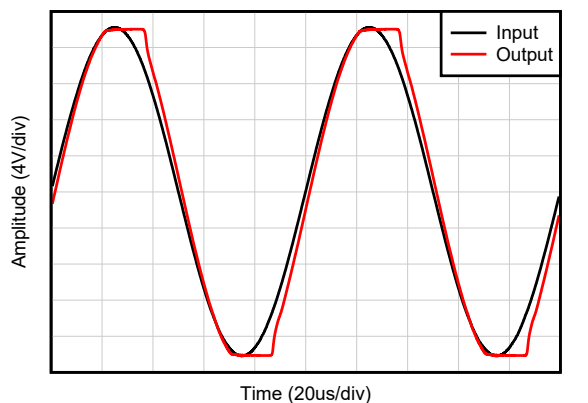
图 7-9. 无相位反转
