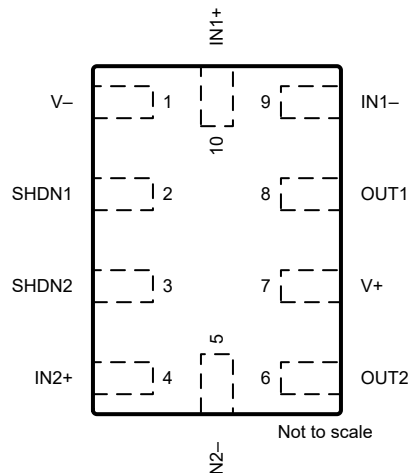
图 5-7. OPA2991S RUG 封装 10 引脚 X2QFN (顶视图)
