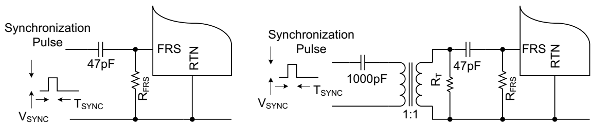
图 7-3. Synchronization
