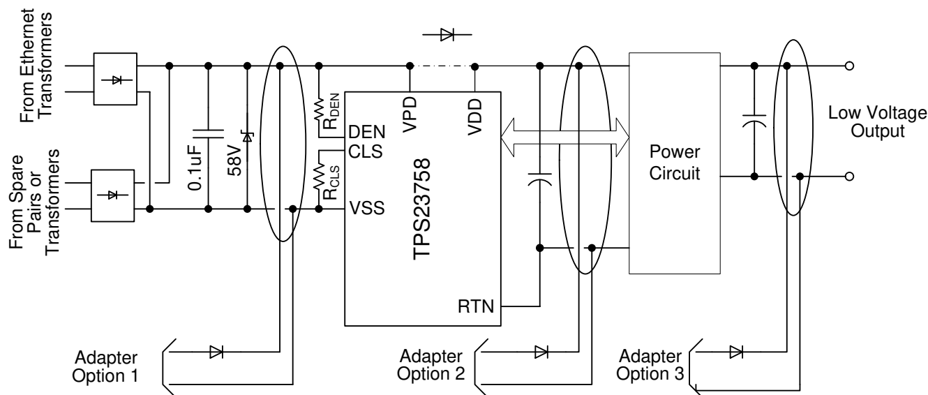
图 7-10. ORing Configurations
