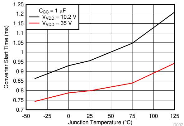
图 6-6. Converter Startup Time vs Temperature
