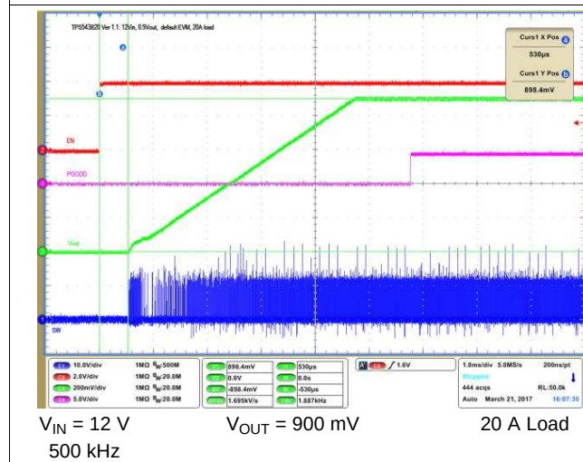
图 11. Start-Up From EN
