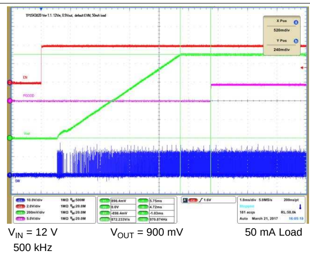
图 10. Startup From EN
