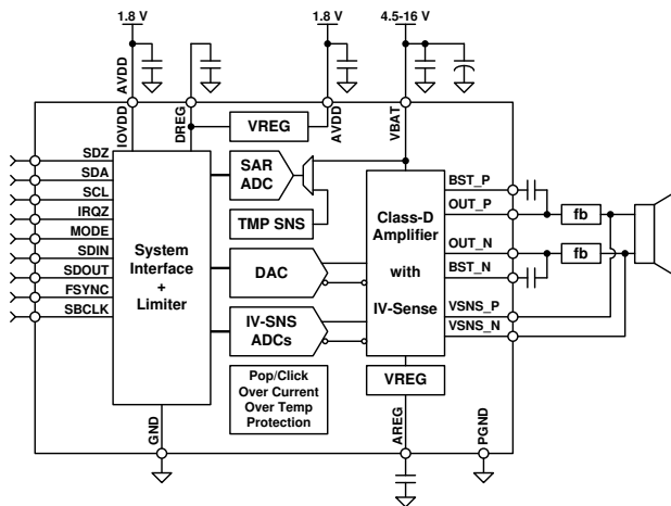
功能方框图
